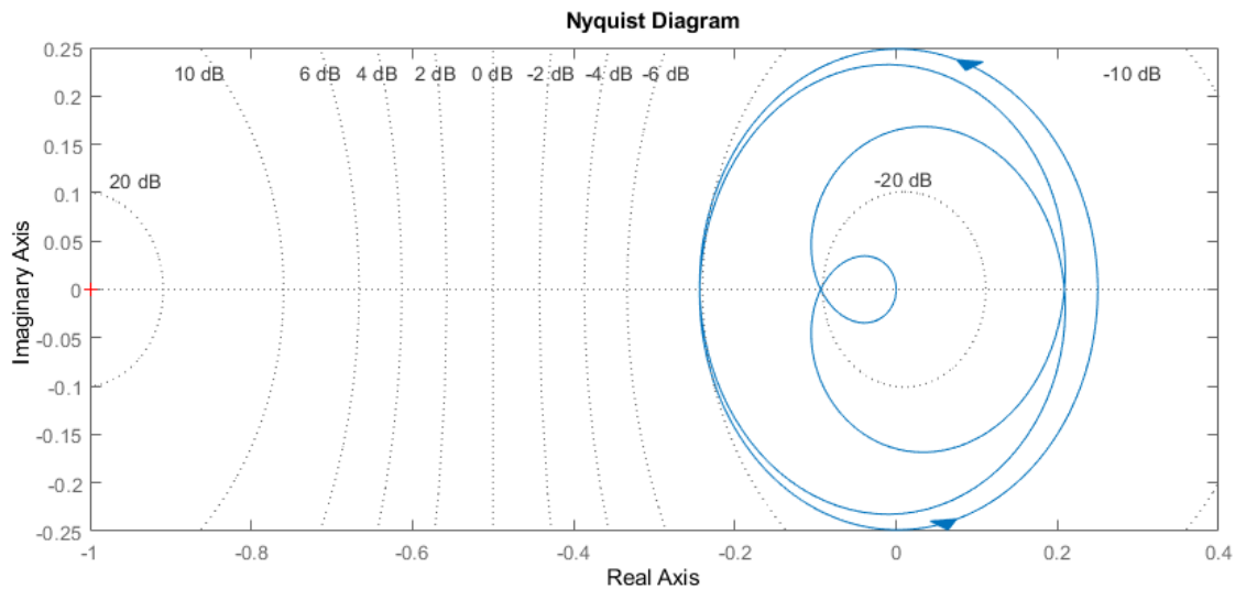
Rysunek 23: Charakterystyka Nyquista dla układu z przykładu 4.
