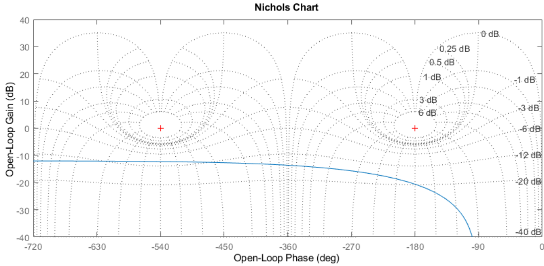
Rysunek 23: Charakterystyka Nicholsa dla układu z przykładu 4.
