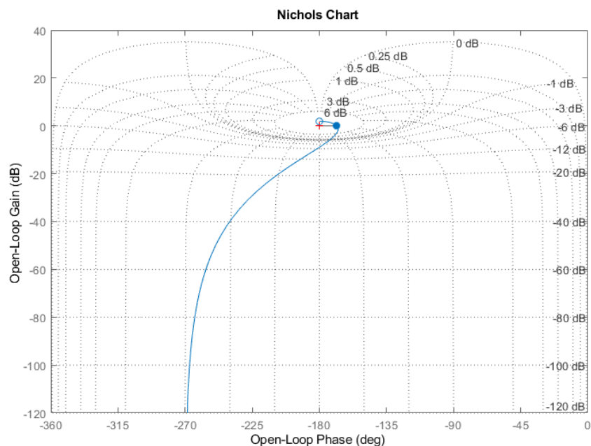
Rysunek 20: Charakterystyka Nicholasa dla układu z przykładu 3.
