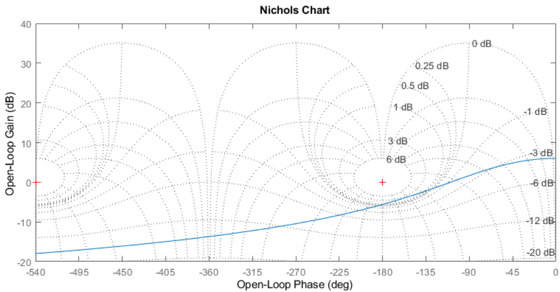
Rysunek 28: Charakterystyka Nicholasa dla układu z przykładu 7.
