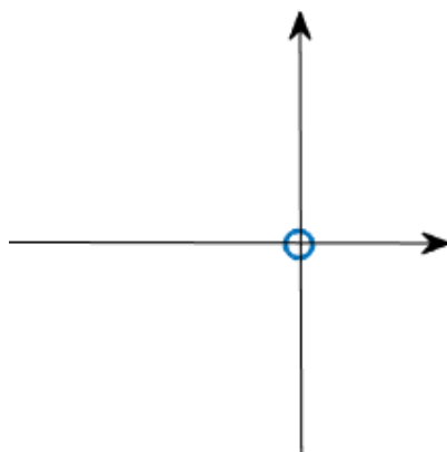
Rysunek 29: Ułożenie wartości własnych dla portretu dla układu z dwoma wartościami własnymi równymi zero i dwoma wektorami własnymi .
