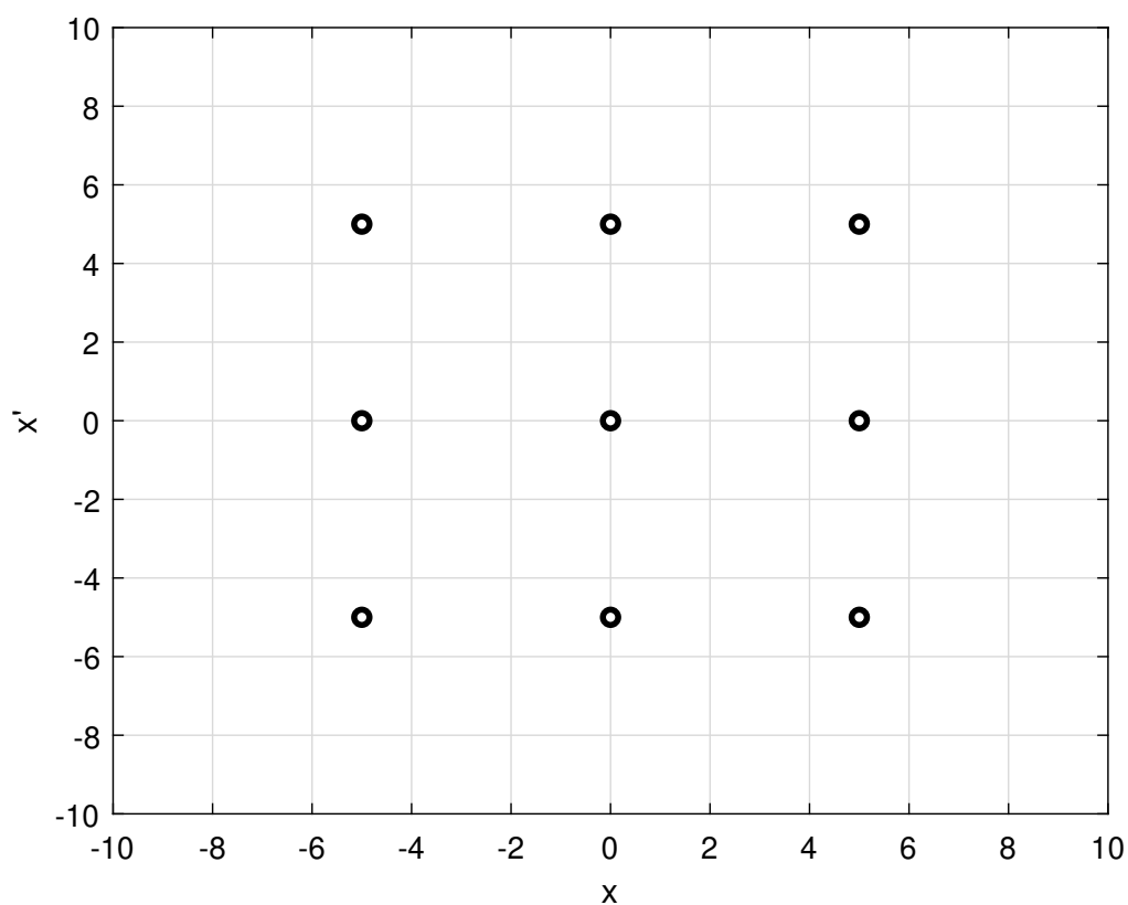
Rysunek 30: Przykładowy portret fazowy dla układu z dwoma wartościami własnymi równymi zero i dwoma wektorami własnymi.
