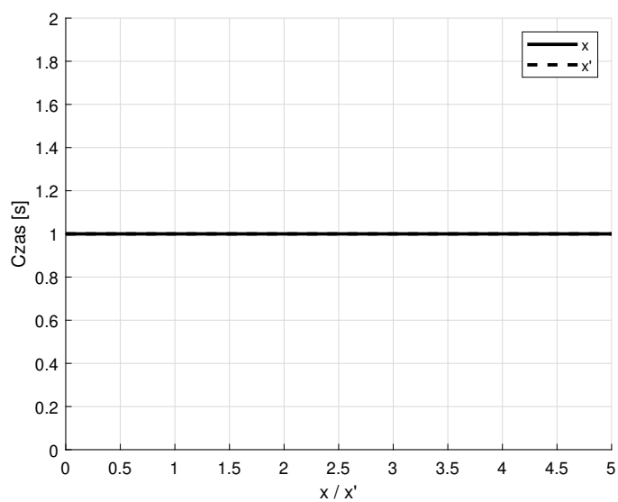
Rysunek 31: Przykładowe przebiegi czasowe dla układu z dwoma wartościami własnymi równymi zero i dwoma wektorami własnymi.
