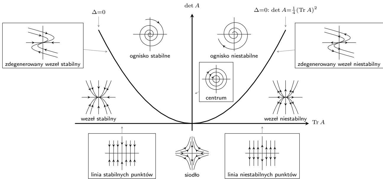
Rysunek 32: Diagram Poincarégo portretów fazowych.
