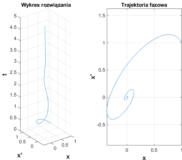
Rysunek 1: Wykres rozwiązania równania (1) i jego trajektoria fazowa.
