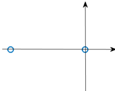
Rysunek 23: Ułożenie wartości własnych dla portretu układów z jednym pierwiastkiem równym 0 .
