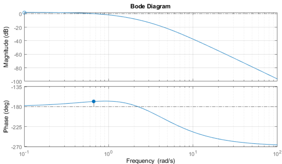
Rysunek 21: Charakterystyka Bodego dla układu z przykładu 3.
