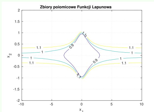
Rysunek 3: Funkcja Lapunowa V(x) jest radialnie ograniczona - zbiór poziomowy dla V(x) = 1 jest niedomknięty.
