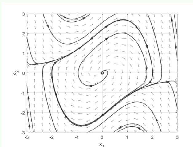
Rysunek 1: Portret fazowy dla oscylatora Van der Pola (równanie 2).
