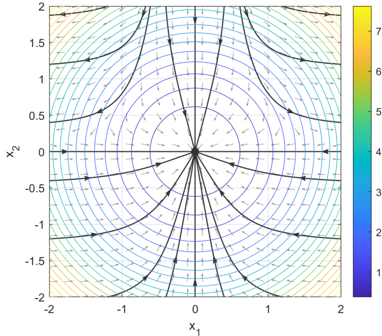
Rysunek 24: Portret fazowy układu (31) z naniesionymi poziomiami funkcji Lapunowa.
