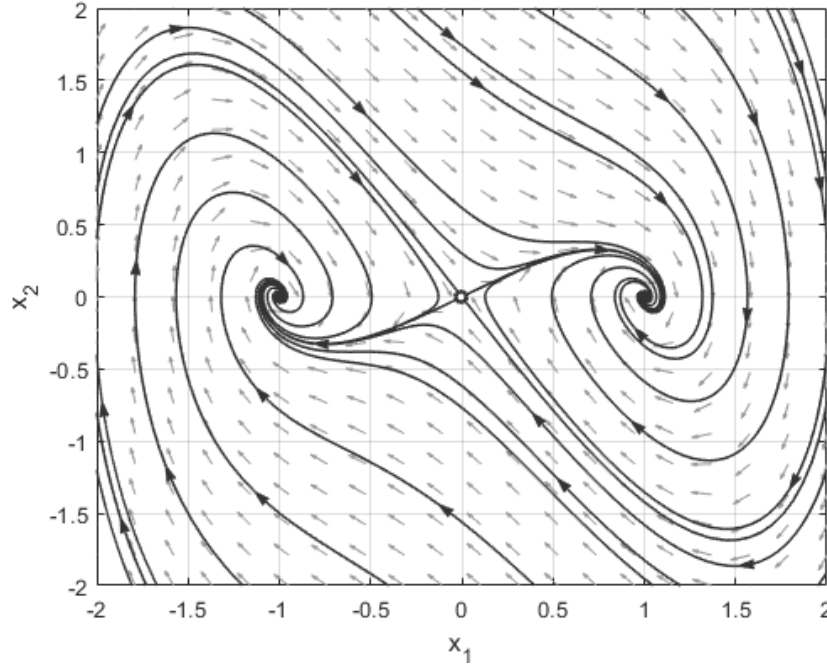
Rysunek 14: Portret fazowy układu (26).
