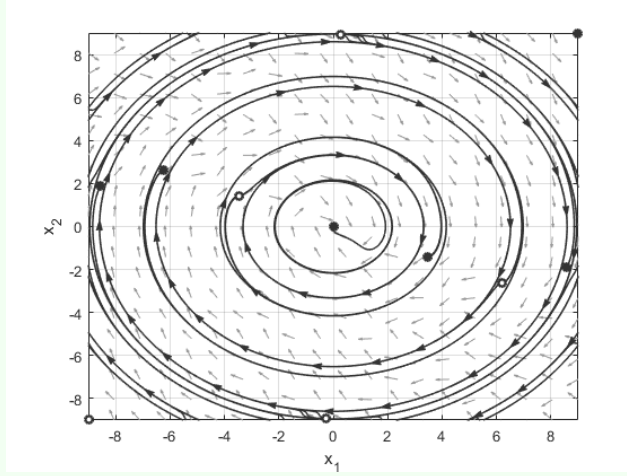
Rysunek 2: Portret fazowy dla układu opisanego układem równań 3.
