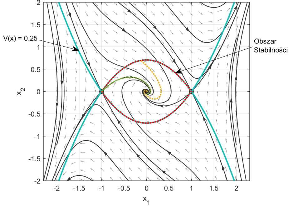
Rysunek 32: Portret fazowy układu (35) z naniesionym obszarem atrakcji stabilnego punktu równowagi (obszar zaznaczony czerwoną przerywaną linią).
