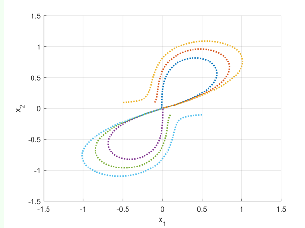
Rysunek 4: Przykładowe trajektorie dla układu (7).
