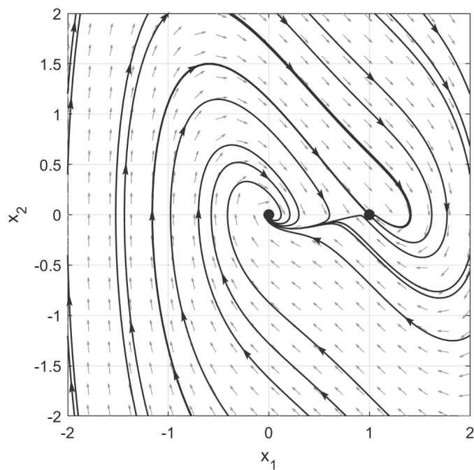
Rysunek 33: Portret fazowy układu (38).
