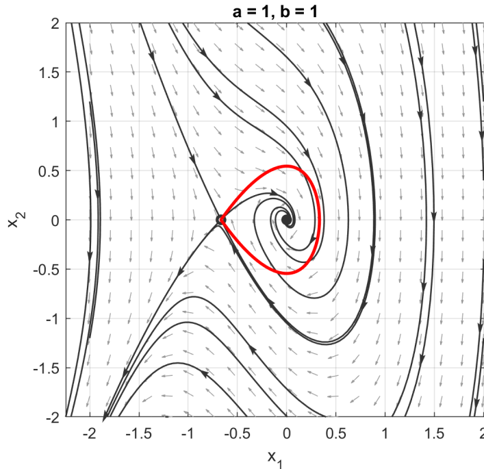
Rysunek 40: Oszacowanie obszaru przyciągania punktu równowagi układu z przykładu 9 dla funkcji Lapunowa w postaci (45). Dla parametrów a = 1 i b = 1 .
