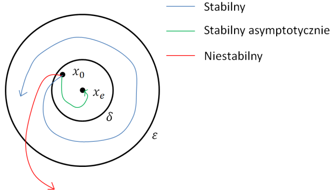
Rysunek 3: Interpretacja geometryczna definicji stabilności.
