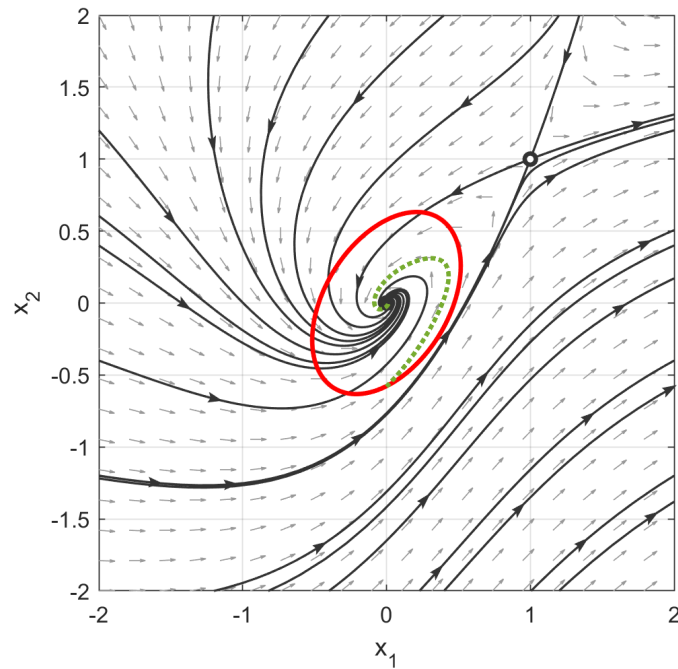
Rysunek 20: Estymata obszaru atrakcji na tle portretu fazowego z przykładu 4.
