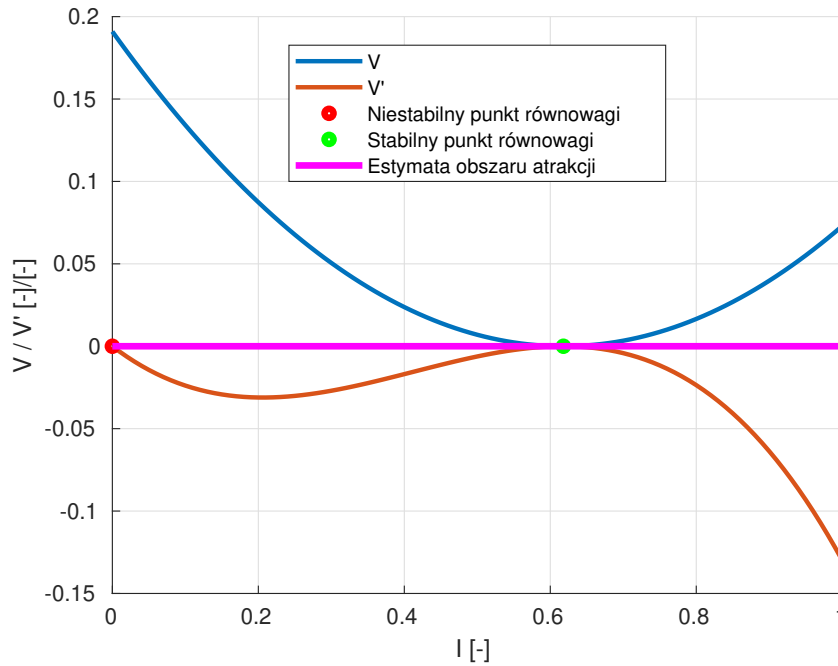
Rysunek 45: Funkcja Lapunowa (53) i jej pochodna systemowa (54) dla modelu SI.
