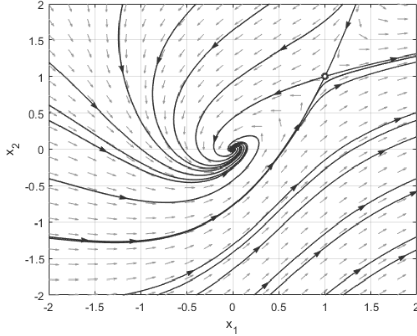
Rysunek 13: Portret trajektorii stanu układu (24).
