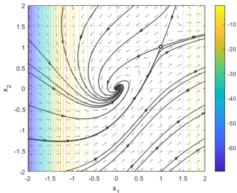
Rysunek 22: Poziomice pochodnej systemowej funkcji Lapunowa (30) na tle portretu fazowego z przykładu 4.
