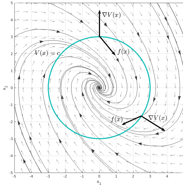
Rysunek 8: Geometryczna interpretacja warunku na inwariantność zbioru poziomowego.
