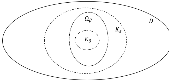
Rysunek 5: Zbiory definiowane w dowodzie twierdzenia Lapunowa o stabilności.
