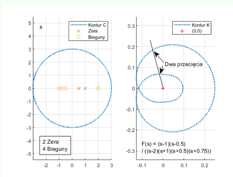
Rysunek 7: Zasada argumentu dla funkcji F(s) = \frac{(s-1)(s-0.5)}{(s-2)(s+0.5)(s+1)(s+0.75)} i konturu zdefiniowanego jako okrąg o promieniu 3 i środkiem w punkcie (0, 0) .
