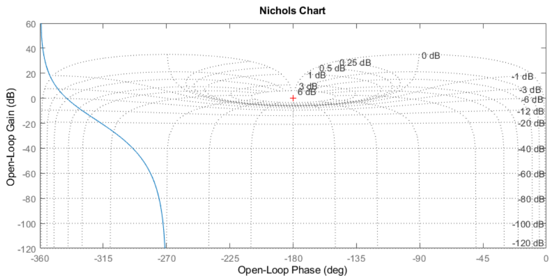
Rysunek 28: Charakterystyka Nicholasa dla układu z przykładu 6.
