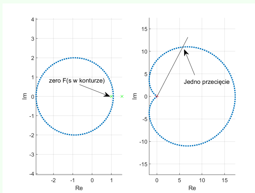
Rysunek 5: Zasada argumentu dla funkcji F(s) = (s - 1)(s - 1.55) i konturu zdefiniowanego jako okrąg o promieniu 2 i środkem w punkcie (-0.9,0).
