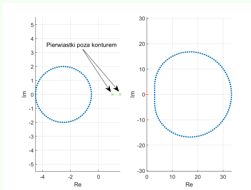
Rysunek 6: Zasada argumentu dla funkcji F(s) = (s - 1)(s - 1.55) i konturu zdefiniowanego jako okrąg o promieniu 2 i środkiem w punkcie (-2.5, 0) .
