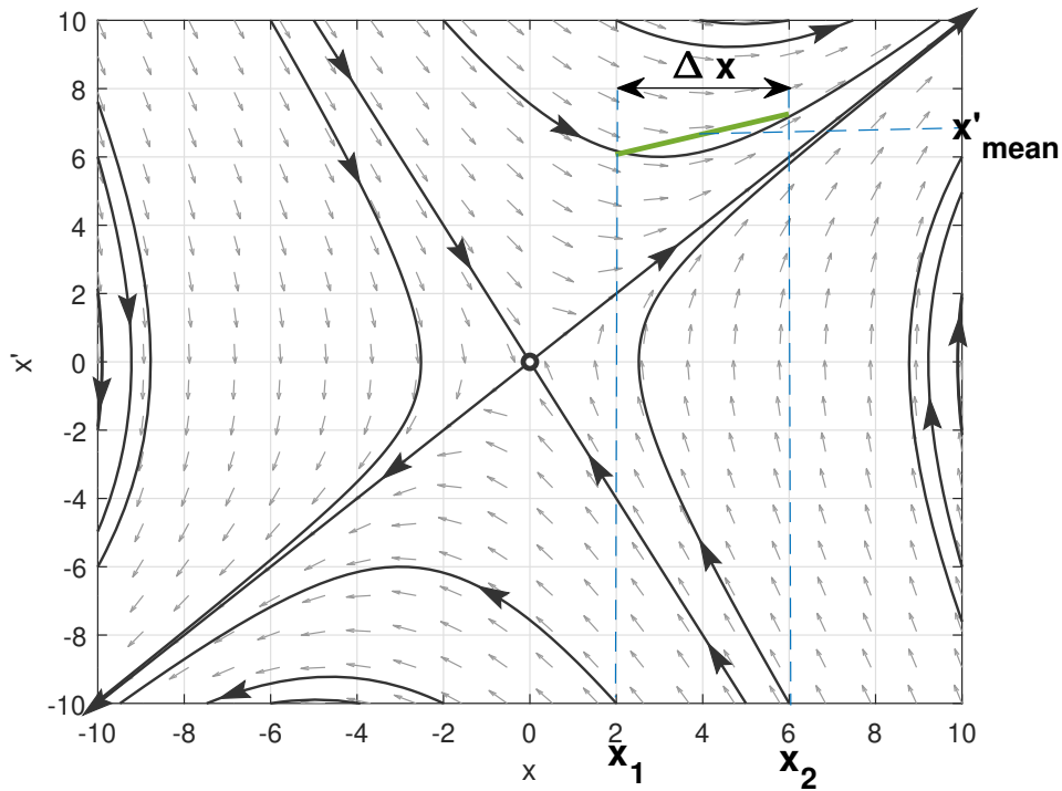
Rysunek 2: Aprosksymacja trajektorii fazowej odcinkami.
