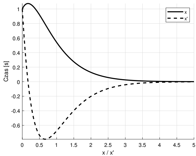
Rysunek 16: Przykładowe przebiegi czasowe dla portretu typu węzeł stabilny .
