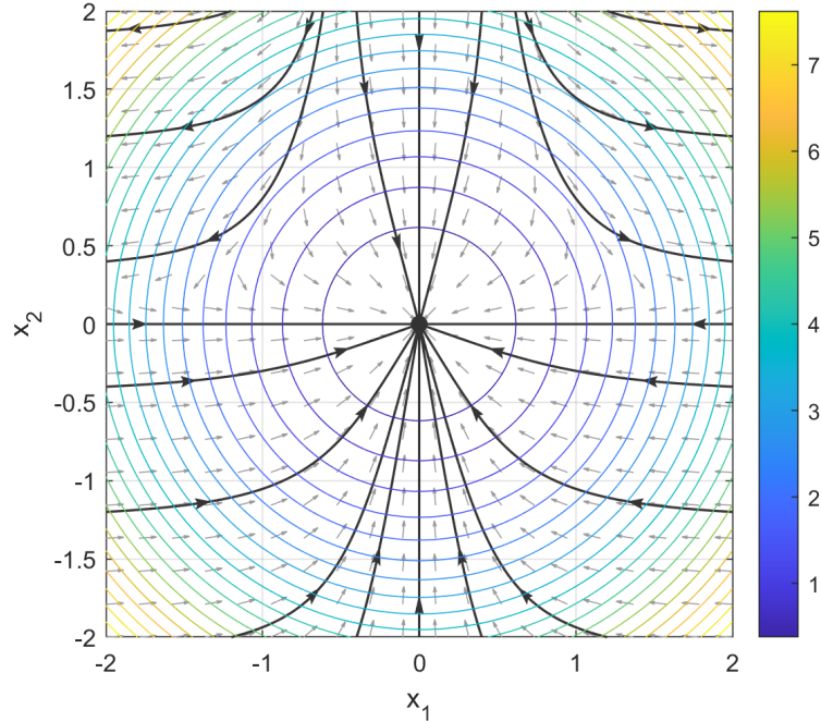
Rysunek 24: Portret fazowy układu (31) z naniesionymi poziomicami funkcji Lapunowa.
