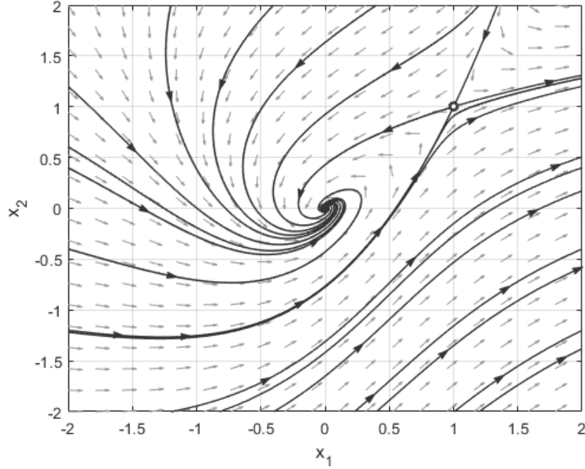
Rysunek 13: Portret trajektorii stanu układu (24).
