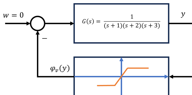
Rysunek 15: Układ sterowania z przykładu 2.
