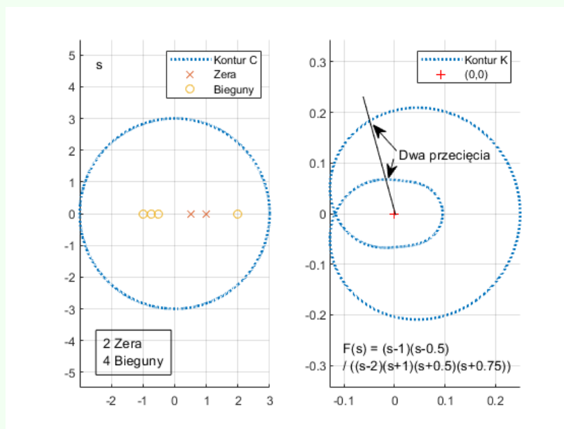
Rysunek 7: Zasada argumentu dla funkcji F(s) = \frac{(s-1)(s-0.5)}{(s-2)(s+0.5)(s+1)(s+0.75)} i konturu zdefiniowanego jako okrąg o promieniu 3 i środku w punkcie (0, 0) .
