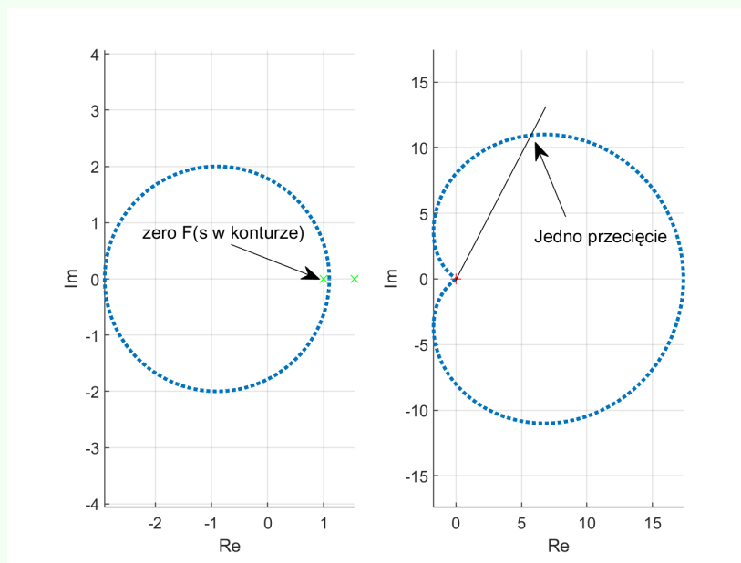
Rysunek 5: Zasada argumentu dla funkcji F(s) = (s - 1)(s - 1.55) i konturu zdefiniowanego jako okrąg o promieniu 2 i środku w punkcie (-0.9,0).
