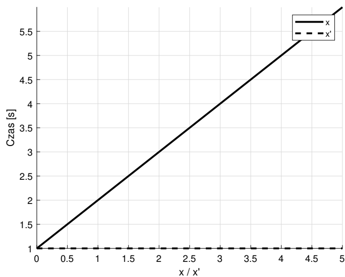
Rysunek 28: Przykładowe przebiegi czasowe dla dwóch pierwiastków równych 0 (z jednym wektorem własnym ).
