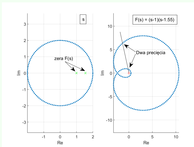
Rysunek 4: Zasada argumentu dla funkcji F(s) = (s - 1)(s - 1.55) i konturu zdefiniowanego jako okrąg o promieniu 2 i środkem w punkcie (0,0).
