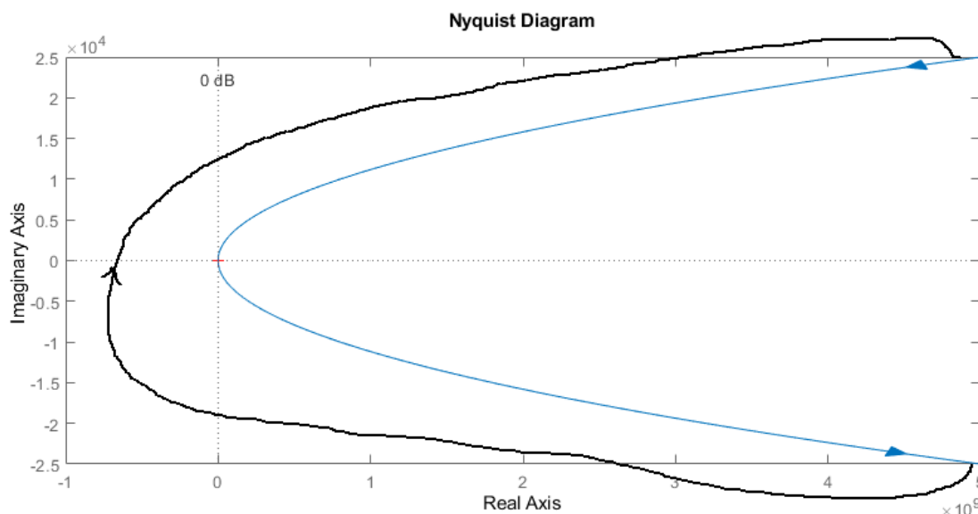
Rysunek 25: Charakterystyka Nyquista dla układu z przykładu 6.
