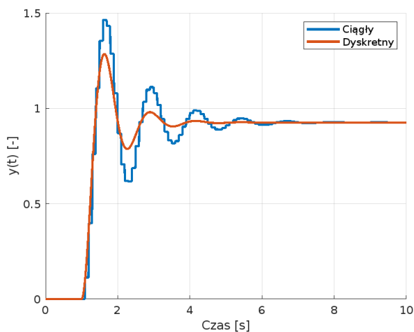
Rysunek 12: Wyjście układu sterowania z czasem ciągłym i dyskretnym dla przykładu 2.
