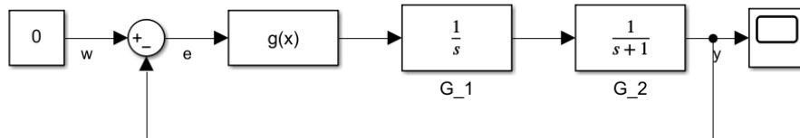
Rysunek 28: Schemat układu regulacji z przykładu 6.
