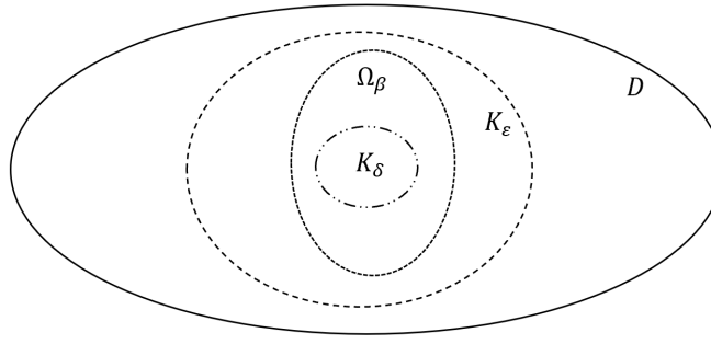
Rysunek 10: Zbiory definiowane w dowodzie twierdzenia Lapunowa o stabilności.
