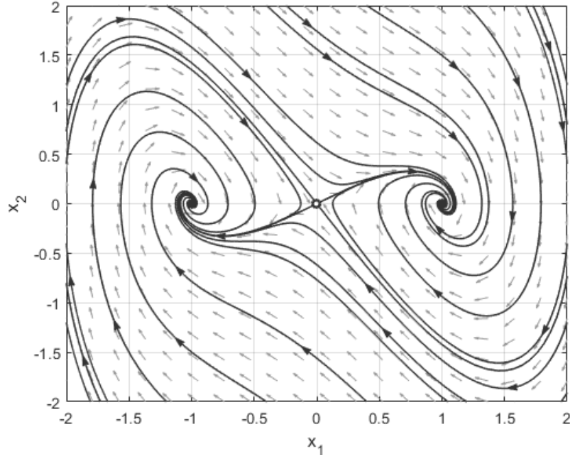
Rysunek 19: Portret fazowy układu (26).
