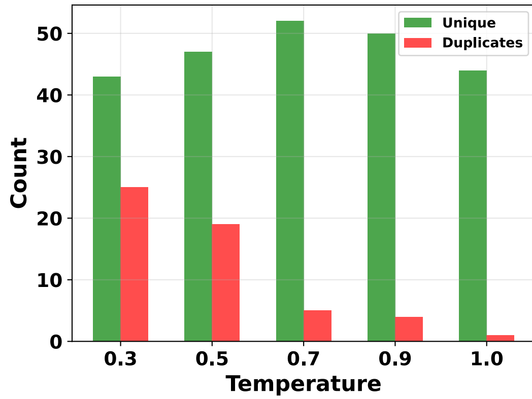
GPT4
