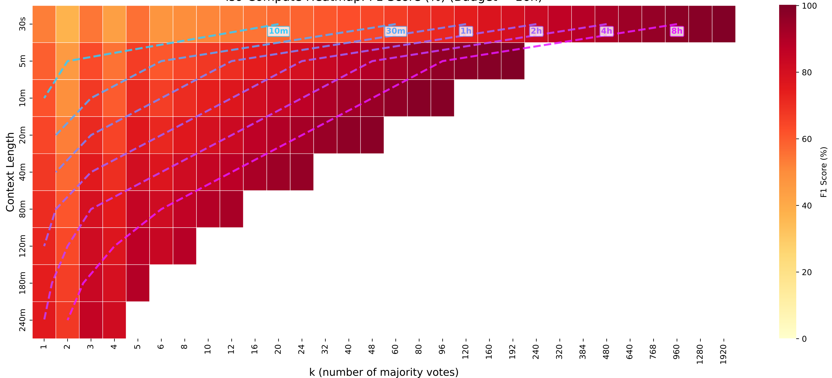
Iso-Compute Heatmap: F1 Score (%) (Budget = 16h)
