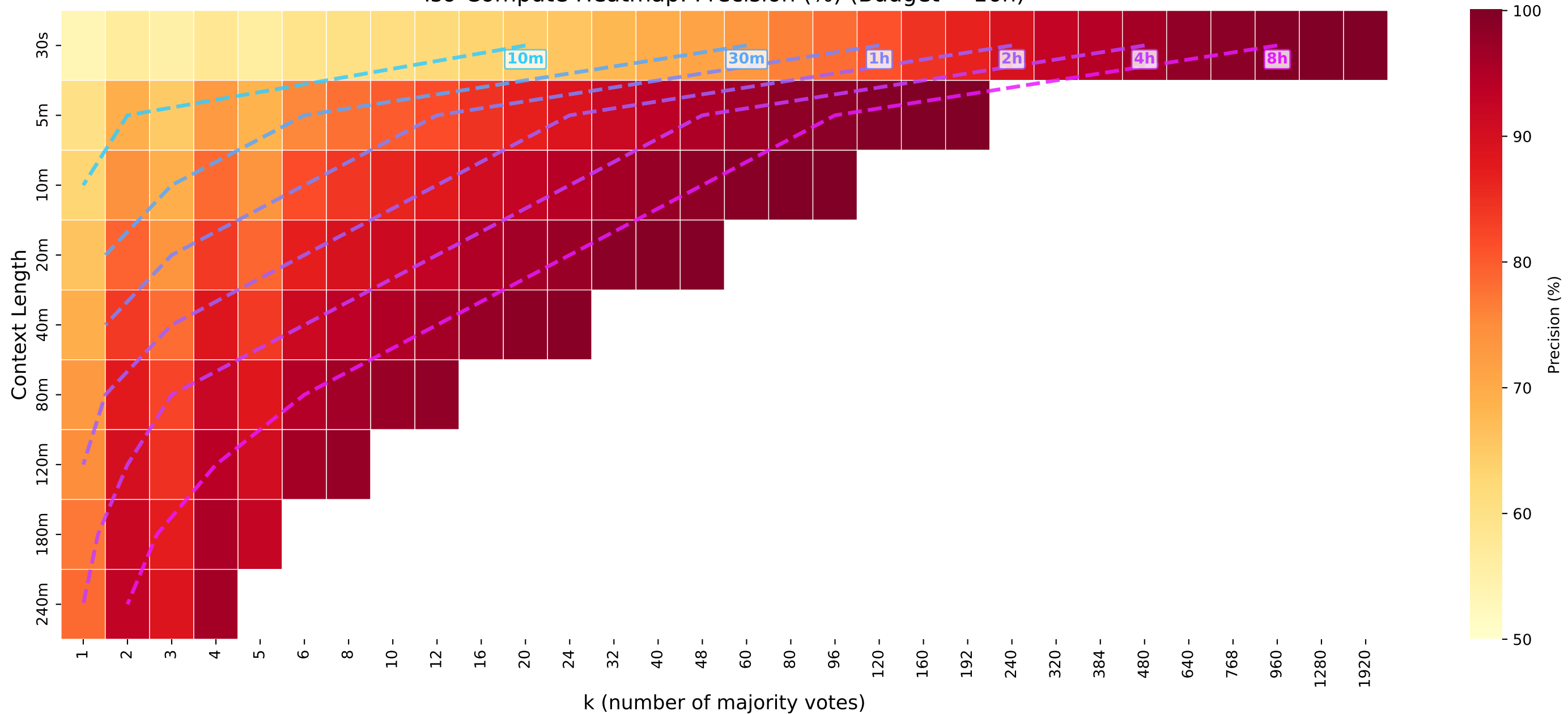
Iso-Compute Heatmap: Precision (%) (Budget = 16h)
