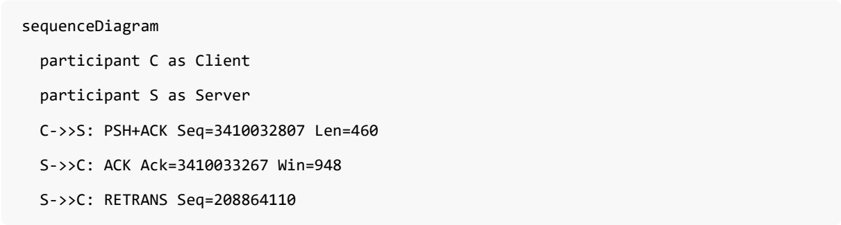
图 3 TCP 数据传输与重传示意
