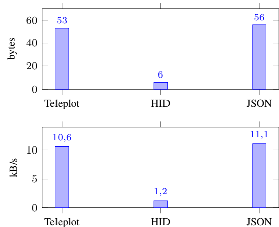
Figura 3. Tamaño de payload (arriba) y ancho de banda a tasa fija de 200 muestras/s (abajo) por protocolo.
