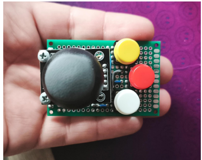
Figura 1. Montaje físico del control: joystick analógico de dos ejes y tres pulsadores soldados sobre una placa perforada.
