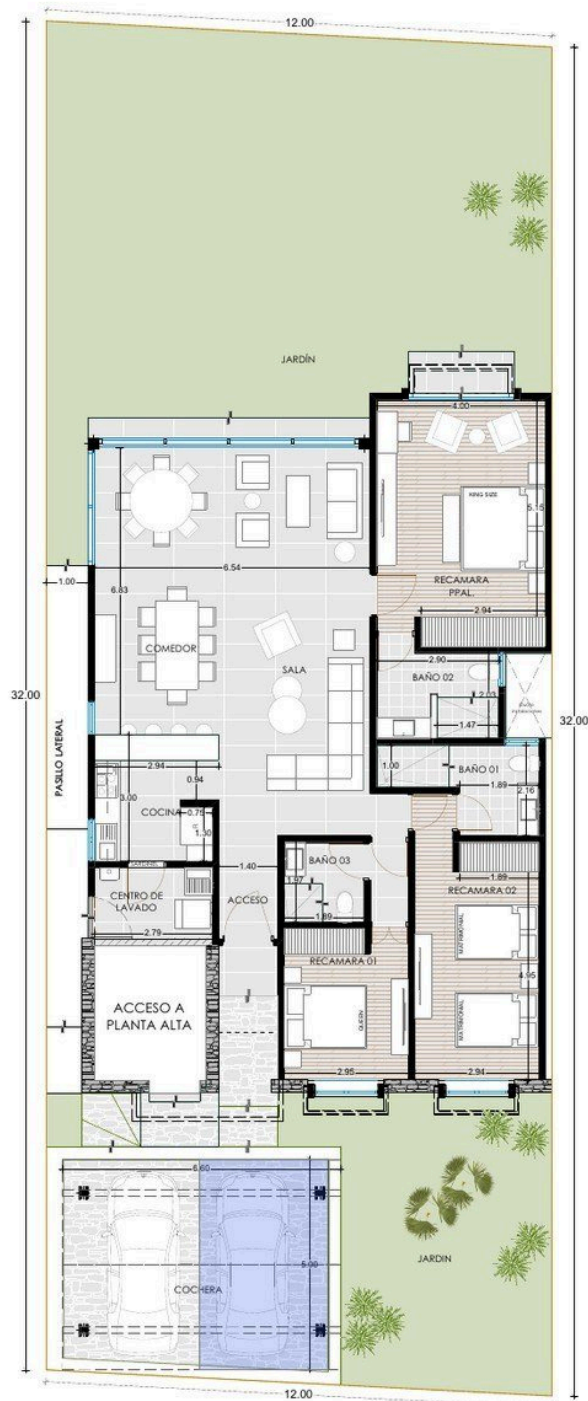
PLANTA BAJA
