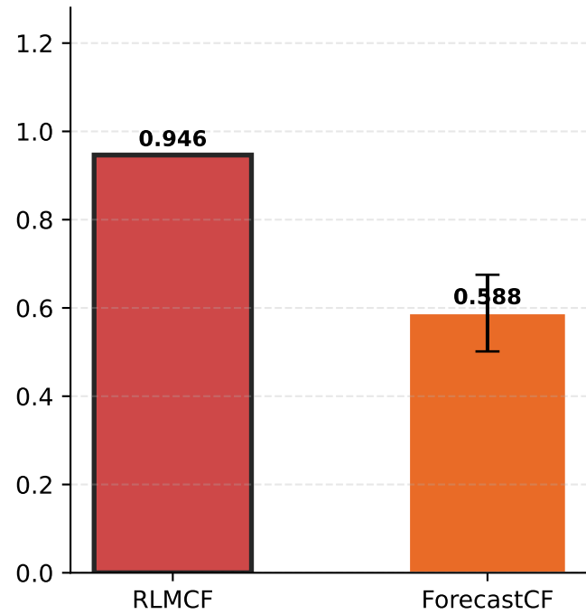
Step AUC ↑
