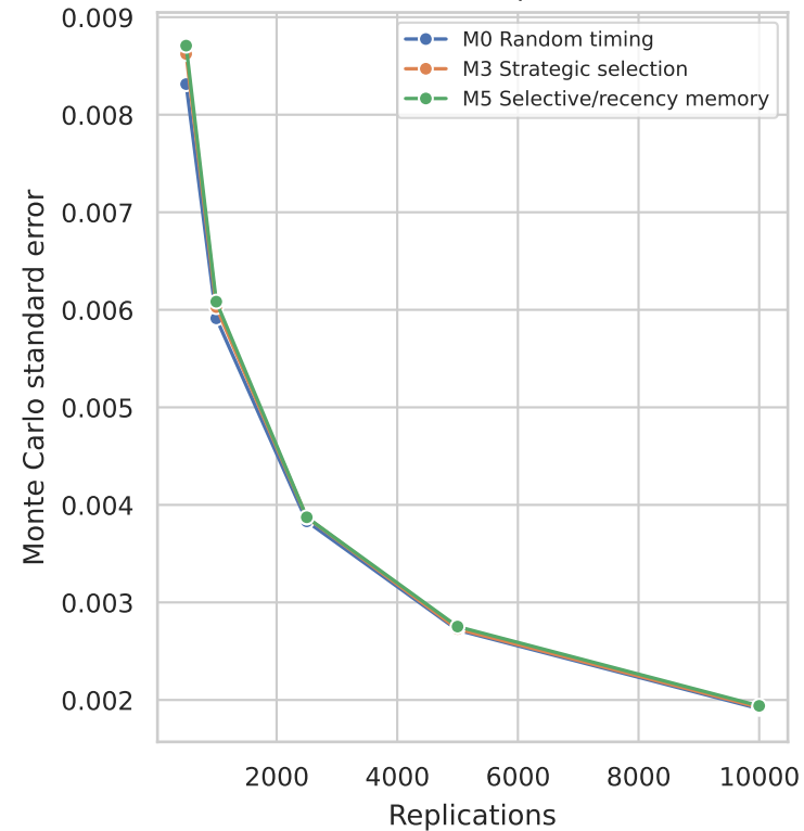
C. Monte Carlo precision
