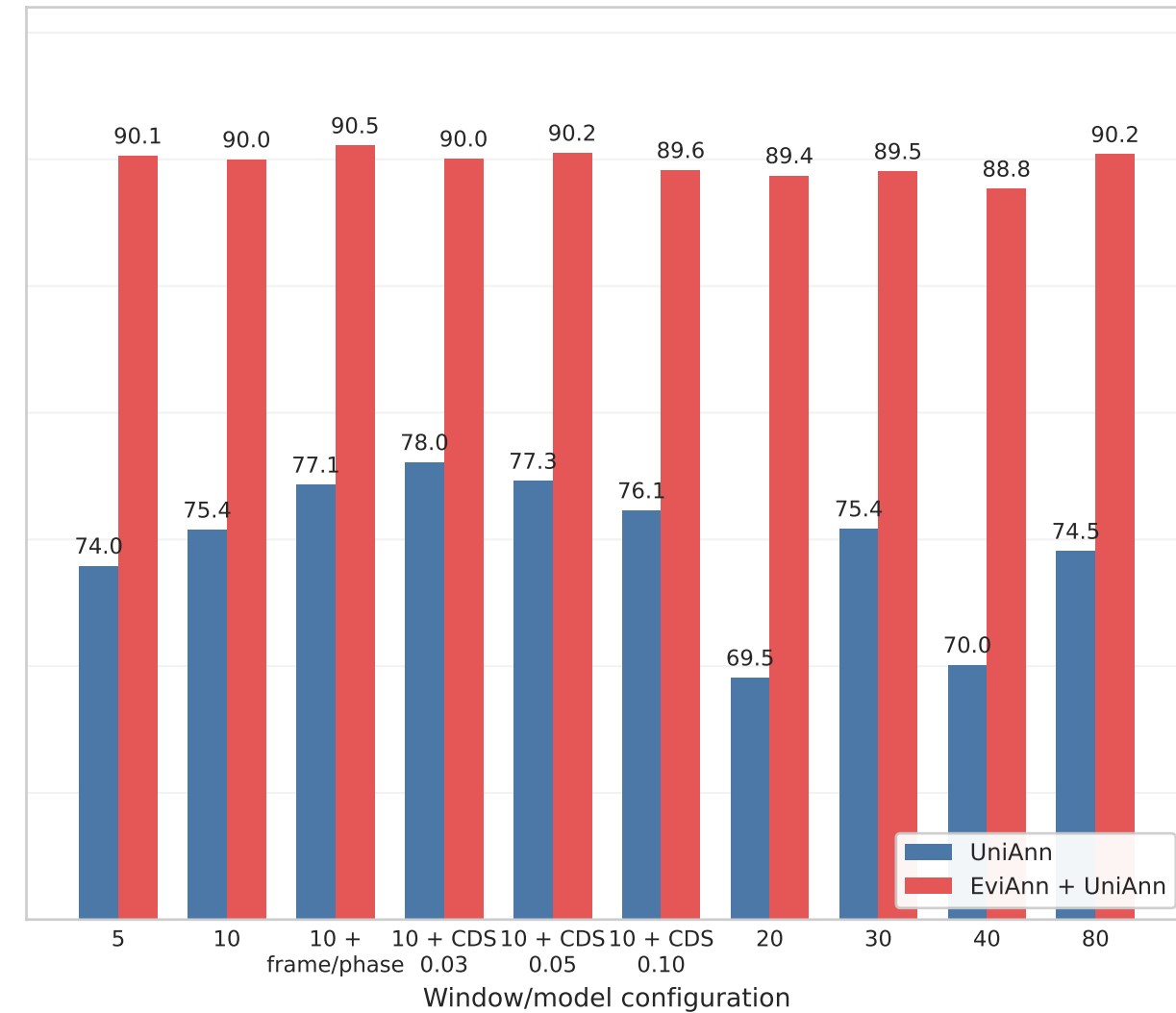
Locus F1
