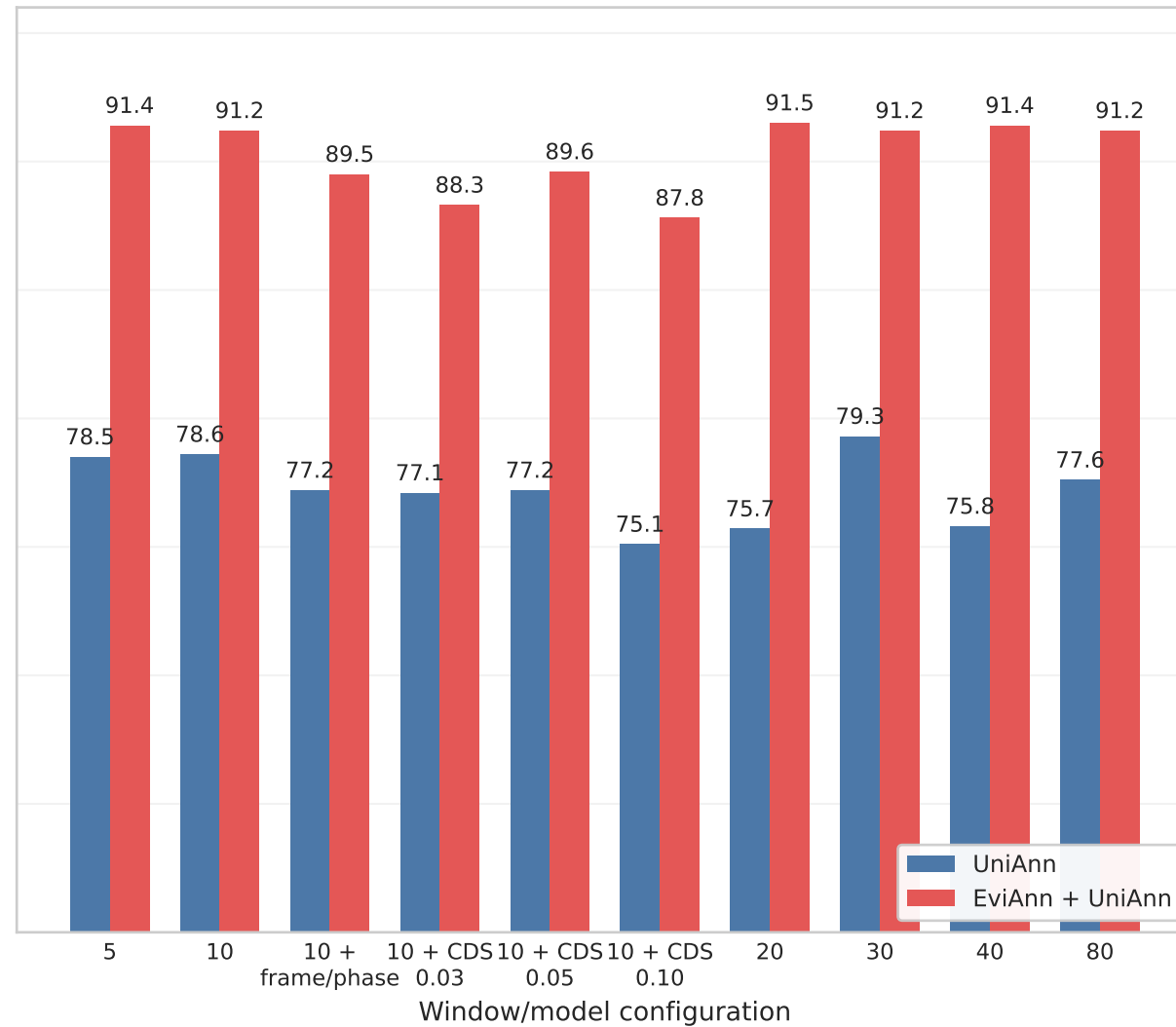
Locus precision
