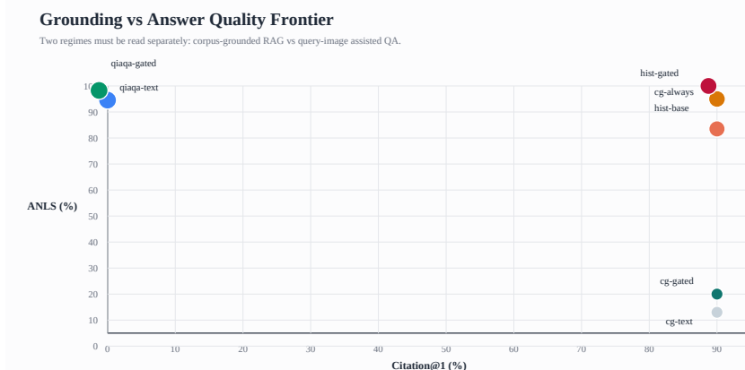
图 2: Grounding 与回答质量的整体权衡。
