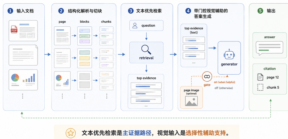
图 1: 系统整体流程图。该流程覆盖数据标准化、页面解析、块级索引、检索重排、视觉辅助生成与评测闭环。
