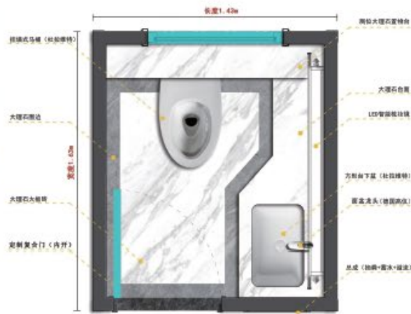
平面布置图
