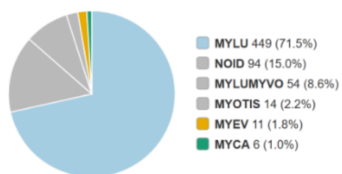
doufr1
