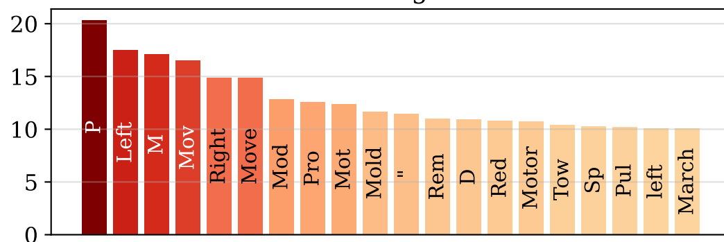
Text logits
