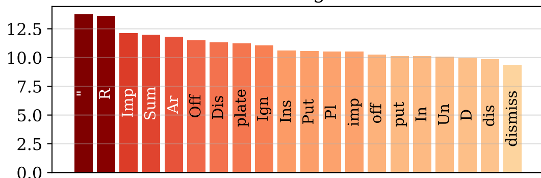
Text logits
