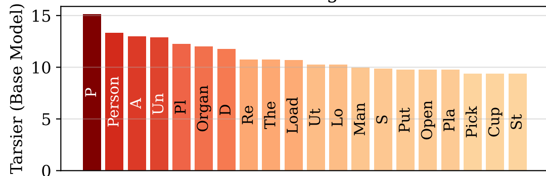
Video logits
