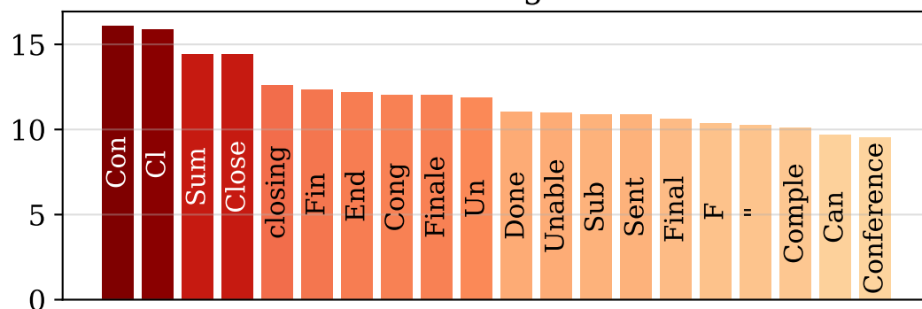
Text logits
