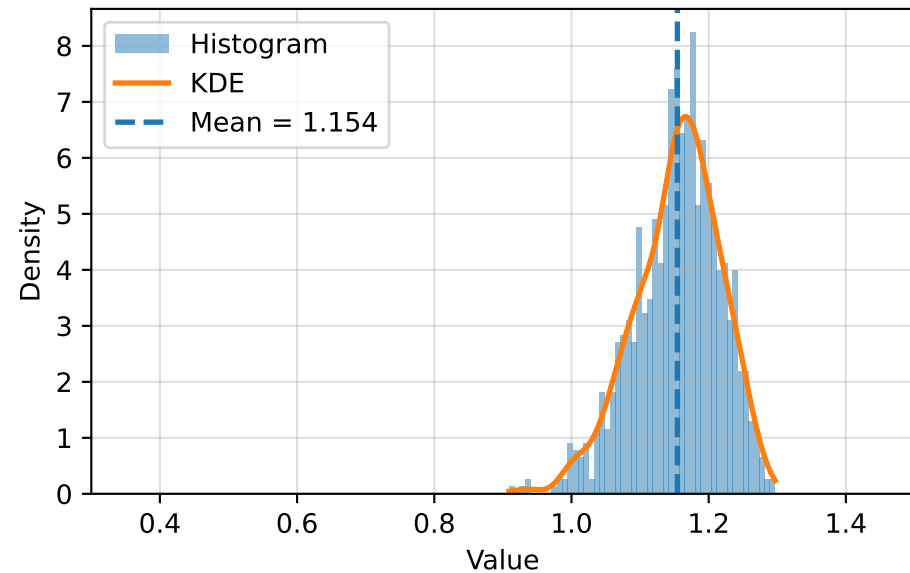
\|g\| (Magnitude)
