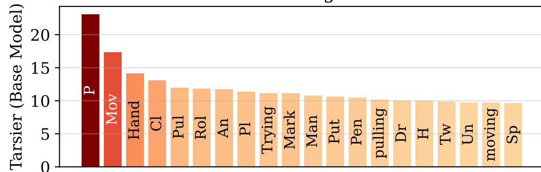
Video logits
