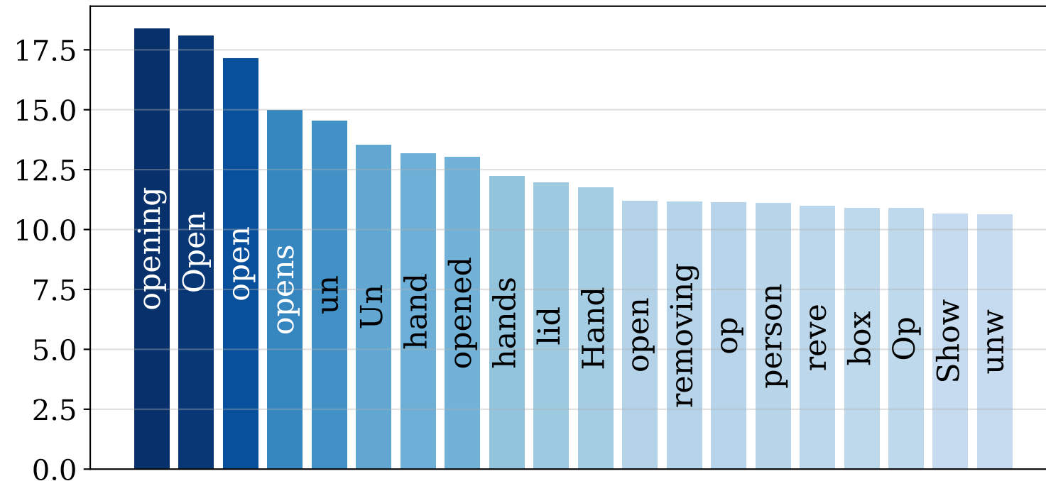
TARA (Ours)
