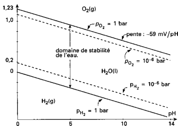
FIGURE 14.2 – Diagramme E-pH de l'eau pour une pression de tracé de 1 bar et de 10^{-6} bar. Source : Université de Batna 2.
