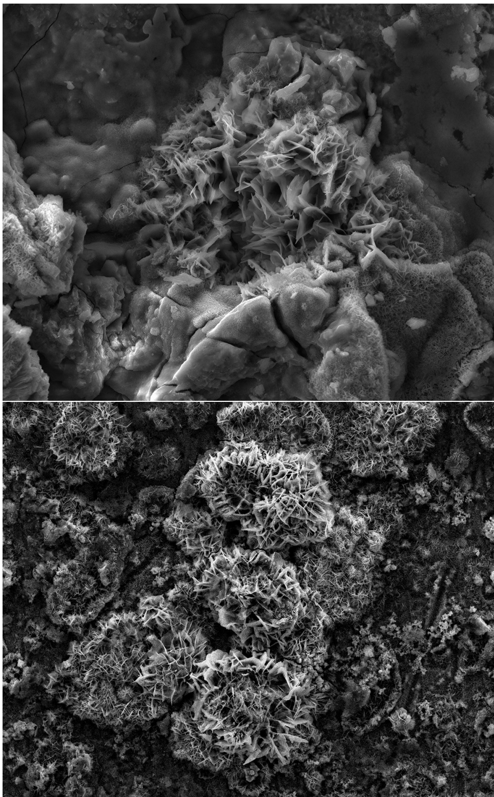
FIGURE 14.4 – Images de plaques de fer corrodées par la pluie (en haut, grossissement \times 3000 ) et l'eau de mer (en bas, grossissement \times 1000 ). Source : Laboratoire des Matériaux et molécules en milieu amazonien, Cayenne.
