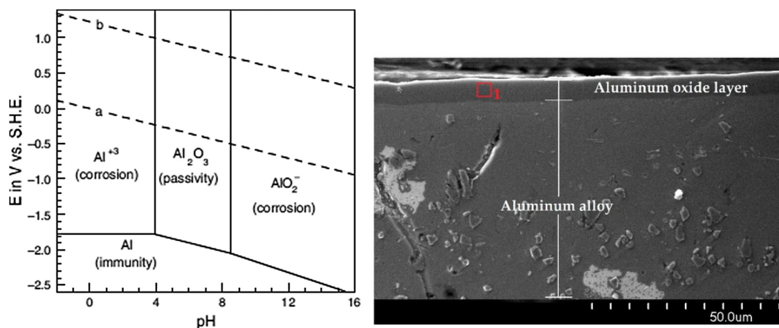
FIGURE 14.3 – A gauche : diagramme potentiel-pH de l'aluminium, avec les domaines d'immunité, de corrosion et de passivation. A droite : Image d'une couche d'oxyde d'aluminium observée au microscope. Sources : Namitha, K., Rao, P., & Rao, S. A. (2022). A brief insight into the use of plant products as green inhibitors for corrosion mitigation of aluminium and aluminium alloys . Canadian Metallurgical Quarterly, 61(4), 429-441. Niedźwiedź, M., Bara, M., Skoneczny, W., Kaptacz, S., & Dercz, G. (2022). Influence of anodizing parameters on tribological properties and wettability of Al 2 O 3 layers produced on the EN AW-5251 aluminum alloy . Materials, 15(21), 7732.
