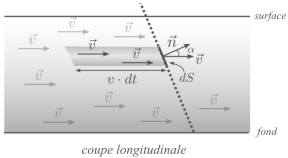
FIGURE 3.11 – Exemple de calcul d'un flux du champ de vitesses à travers la section d'une rivière pour mesurer un débit (cf encart). a) Schéma général de la situation. b) Situation lorsque la surface est perpendiculaire à l'écoulement. c) et d) situation générale. Les images sont reproduites du poly de cours de Daniel Buskulic.
