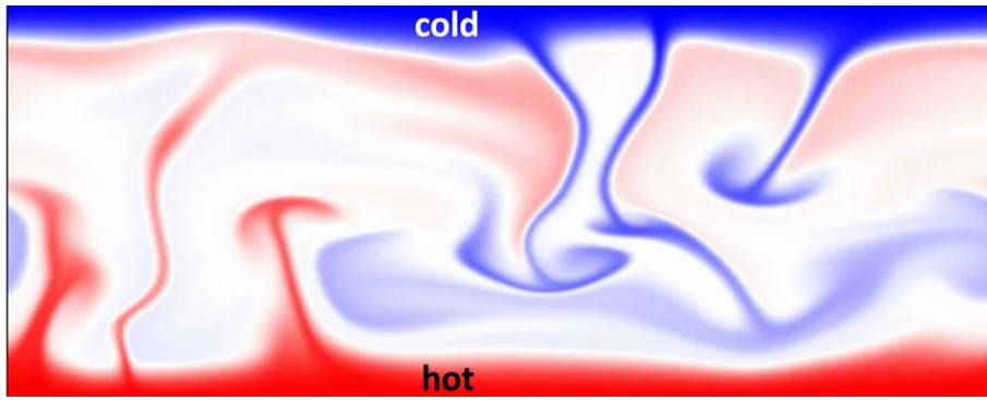
FIGURE 9.3 – Simulation numérique de la convection dans un fluide chauffé par le bas (par exemple, cela pourrait être de l’eau dans une casserole). Les zones rouges indiquent des panaches chaudes ascendantes, et les zones bleues des panaches froides descendantes. Source : Doering, C. R. (2020). Turning up the heat in turbulent thermal convection . Proceedings of the National Academy of Sciences.
