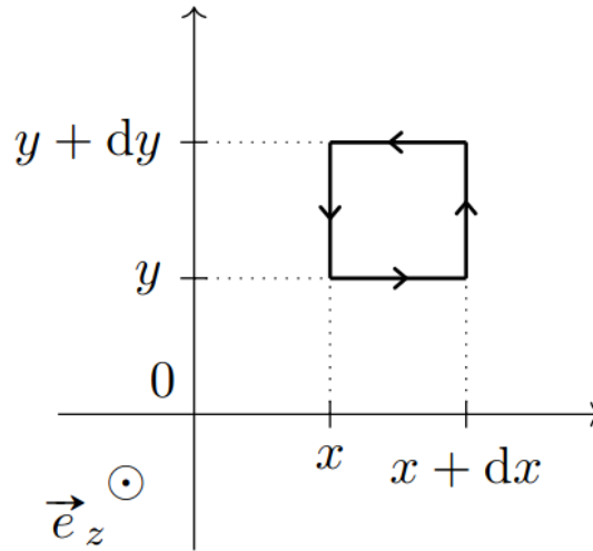
FIGURE 17.3 – Contour mésoscopique utilisé pour calculer la circulation du champ magnétique. Source : poly de cours de Maxime Champion.
