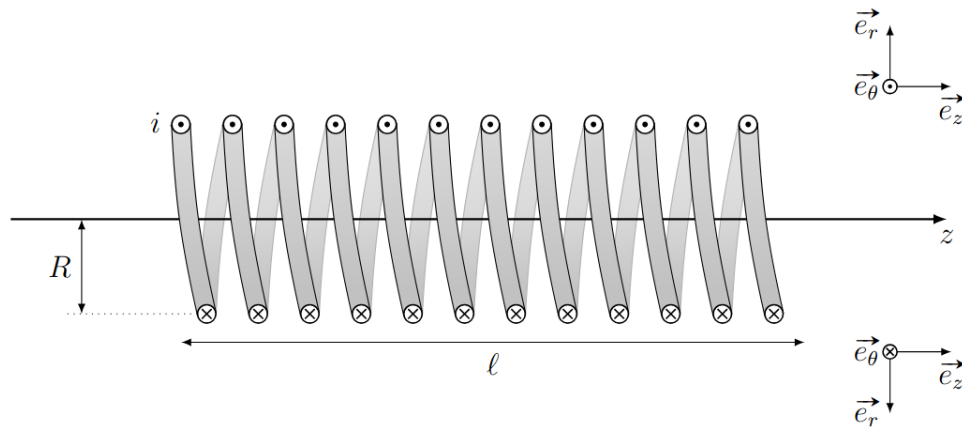
FIGURE 17.8 – Le solénoïde infini
