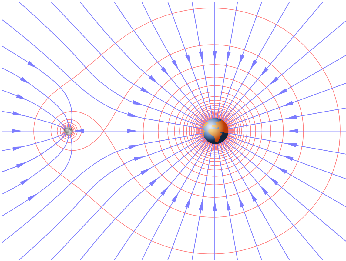
Figure 1.4: Lignes de champ et équipotentielle du système Terre-Lune, qui peuvent être calculées via le principe de superposition. Le champ de gravité est plus fort là où les équipotentielle et les lignes de champ sont les plus resserrées. Le champ est le gradient du potentiel, ainsi les lignes de champ et les équipotentielle sont en tout point perpendiculaires. Source : Wikimedia Commons.
