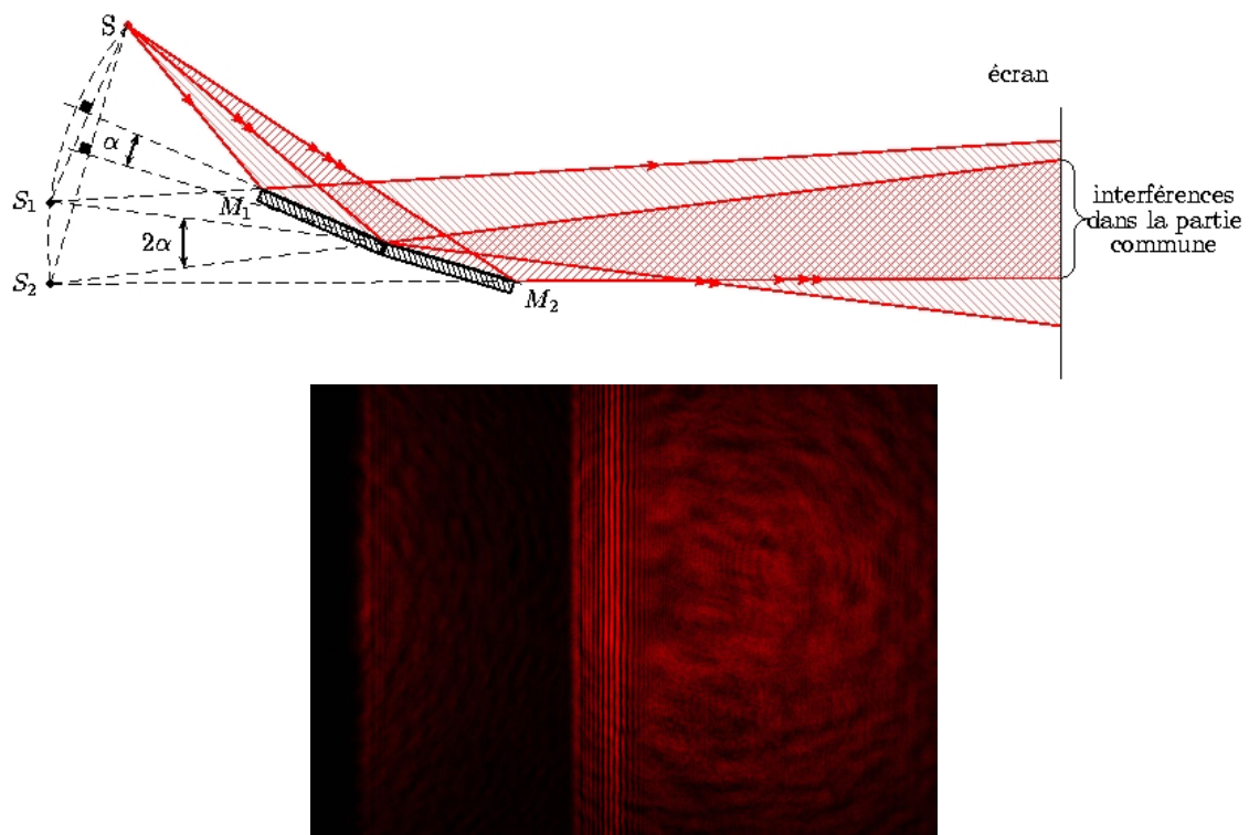
FIGURE 8.6 – Les miroirs de Fresnel. En haut : schéma du dispositif. En bas : photo des interférences observées. Sources : melusine.eu.org et Leybold.
