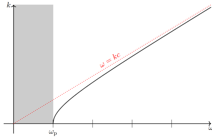
FIGURE 17.6 – Relation de dispersion pour une onde propagative dans un plasma. On constate que la région \omega < \omega_p est interdite. Source : poly de cours de Maxime Champion.
