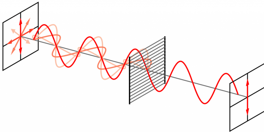
FIGURE 17.4 – Fonctionnement d’un polariseur. La lumière non polarisée est convertie en lumière polarisée (avec absorption d’énergie au niveau du polariseur). Source : Wikimedia Commons.
