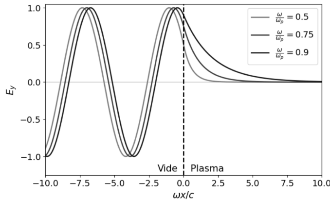
FIGURE 17.7 – Structure d'une onde plane progressive harmonique arrivant à l'interface avec un plasma, pour différentes valeurs de pulsations. L'onde évanescente est visible dans le plasma.
