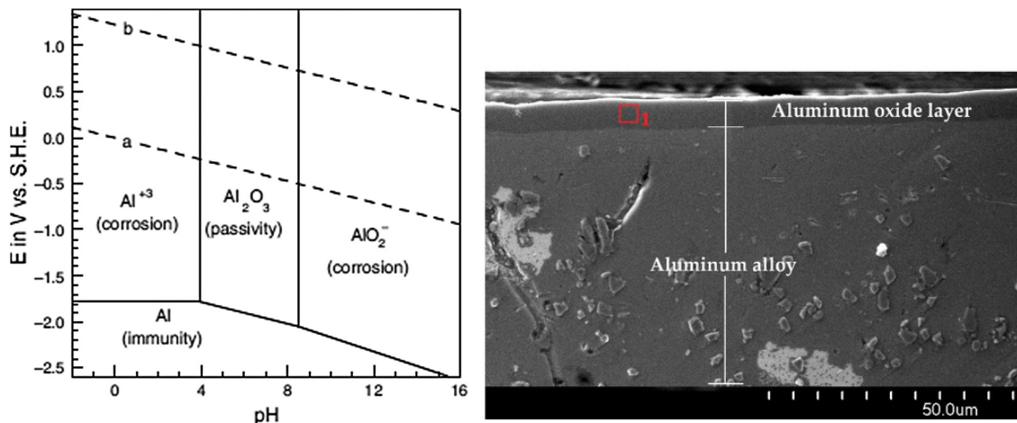
FIGURE 14.5 – A gauche : diagramme potentiel-pH de l'aluminium, avec les domaines d'immunité, de corrosion et de passivation. A droite : Image d'une couche d'oxyde d'aluminium observée au microscope. Sources : Namitha, K., Rao, P., & Rao, S. A. (2022). A brief insight into the use of plant products as green inhibitors for corrosion mitigation of aluminium and aluminium alloys . Canadian Metallurgical Quarterly, 61(4), 429-441. Niedźwiedź, M., Bara, M., Skoneczny, W., Kaptacz, S., & Dercz, G. (2022). Influence of anodizing parameters on tribological properties and wettability of \text{Al}_2\text{O}_3 layers produced on the EN AW-5251 aluminum alloy . Materials, 15(21), 7732.
