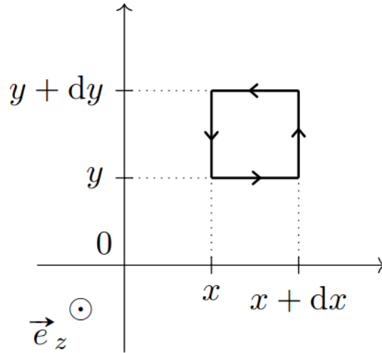
FIGURE 17.2 – Contour mésoscopique utilisé pour calculer la circulation du champ magnétique. Source : poly de cours de Maxime Champion.
