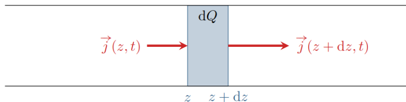
FIGURE 17.3 – Schéma pour le bilan de charge à une dimension. Source : poly de cours de Etienne Thibierge.
