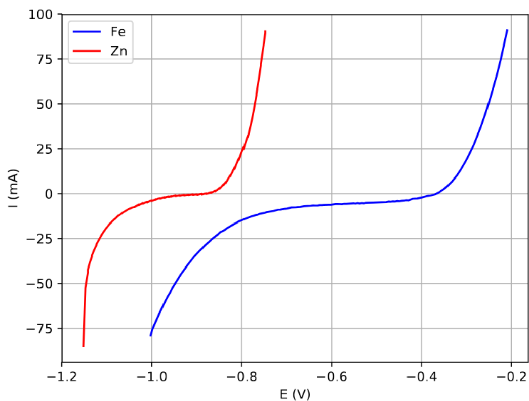
FIGURE 14.8 – Courbes courant-potential obtenues expérimentalement dans de l'eau sur une électrode de fer et une électrode de zinc. Source : poly de TP de Frédéric Legrand.
