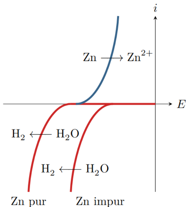
FIGURE 14.6 – Courbes courant-potentiel associées à la corrosion du zinc pur et impur. Source : poly de cours de Etienne Thibierge.
