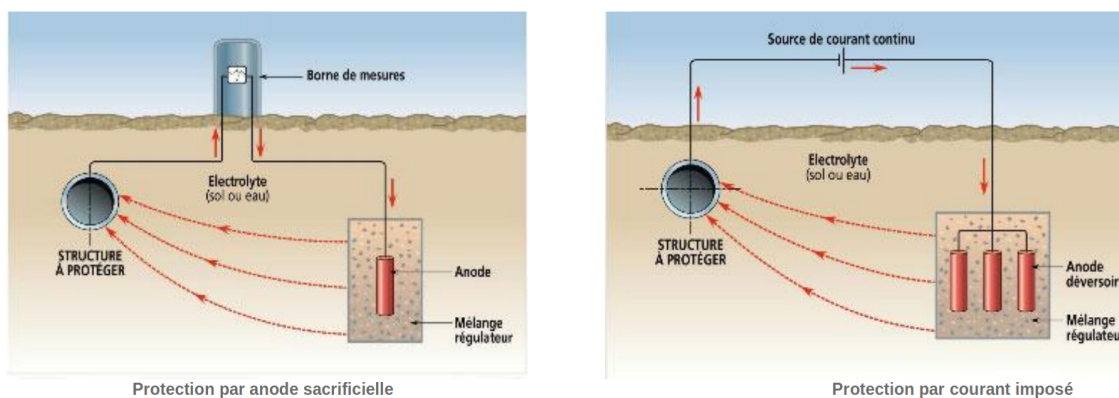
FIGURE 14.11 – Protection d'une canalisation par anode sacrificielle et par courant imposé. Source : poly de cours de Alain Favier.
