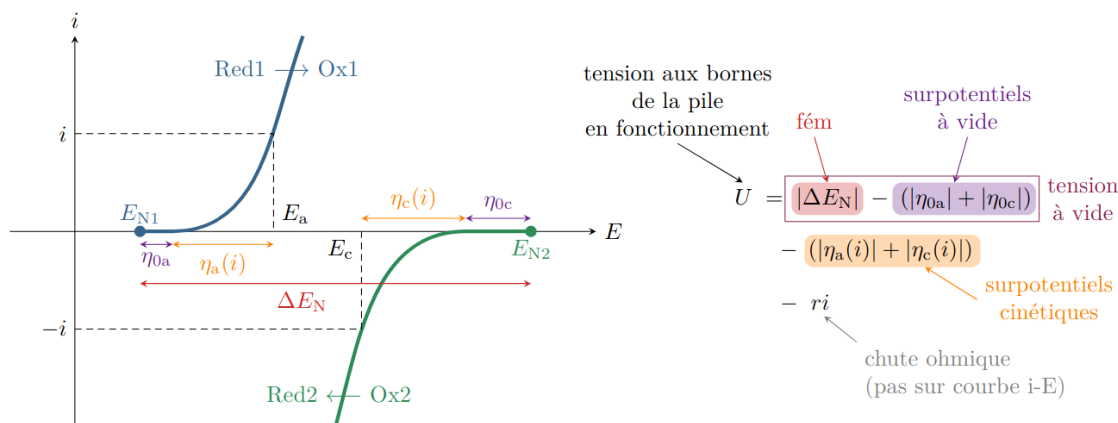
FIGURE 14.12 – Courbes courant-potentiel associées à une pile et différentes sources de la chute de tension. Source : poly de cours de Etienne Thibierge.
