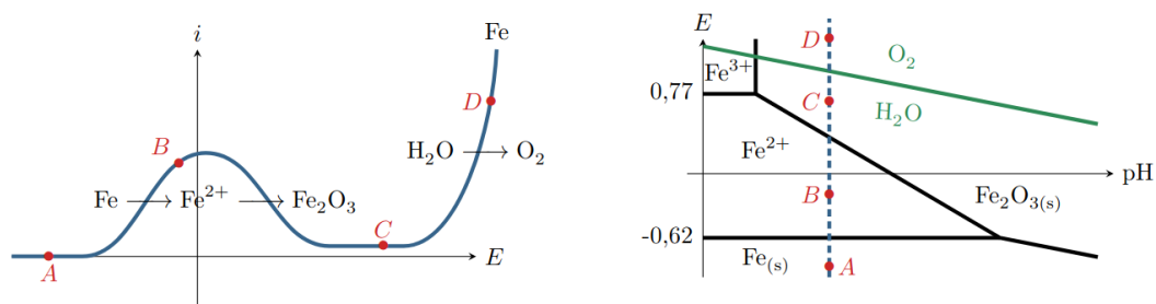
FIGURE 14.7 – Courbes courant-potentiel associées à la corrosion du fer. Source : poly de cours de Etienne Thibierge.
