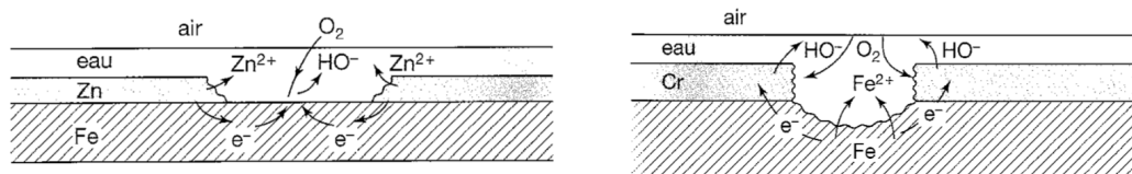
FIGURE 14.10 – Evolution d'un échantillon de fer protégé par un revêtement de zinc (à gauche) et de chrome (à droite), au niveau d'une rayure dans le revêtement. Une pile de corrosion se forme, dont la polarité est inversée dans les deux cas.
