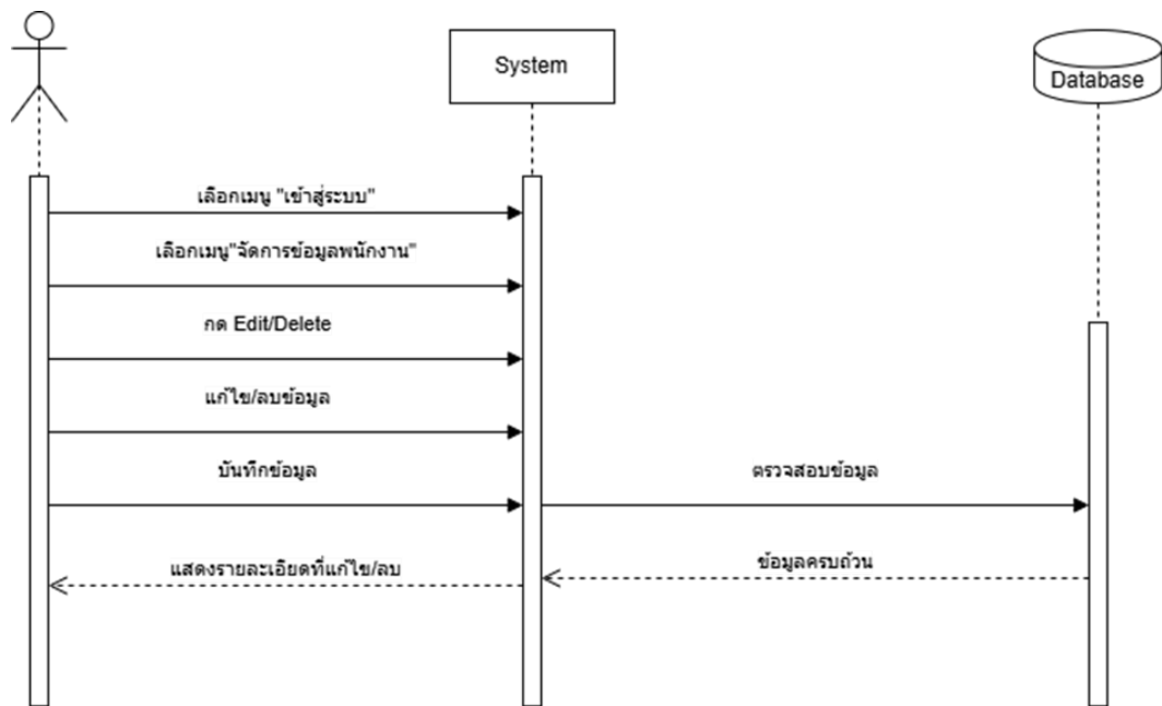
ภาพที่ 19 Sequence Diagram (UC-05) Manage Employee Information (Edit/Delete)
