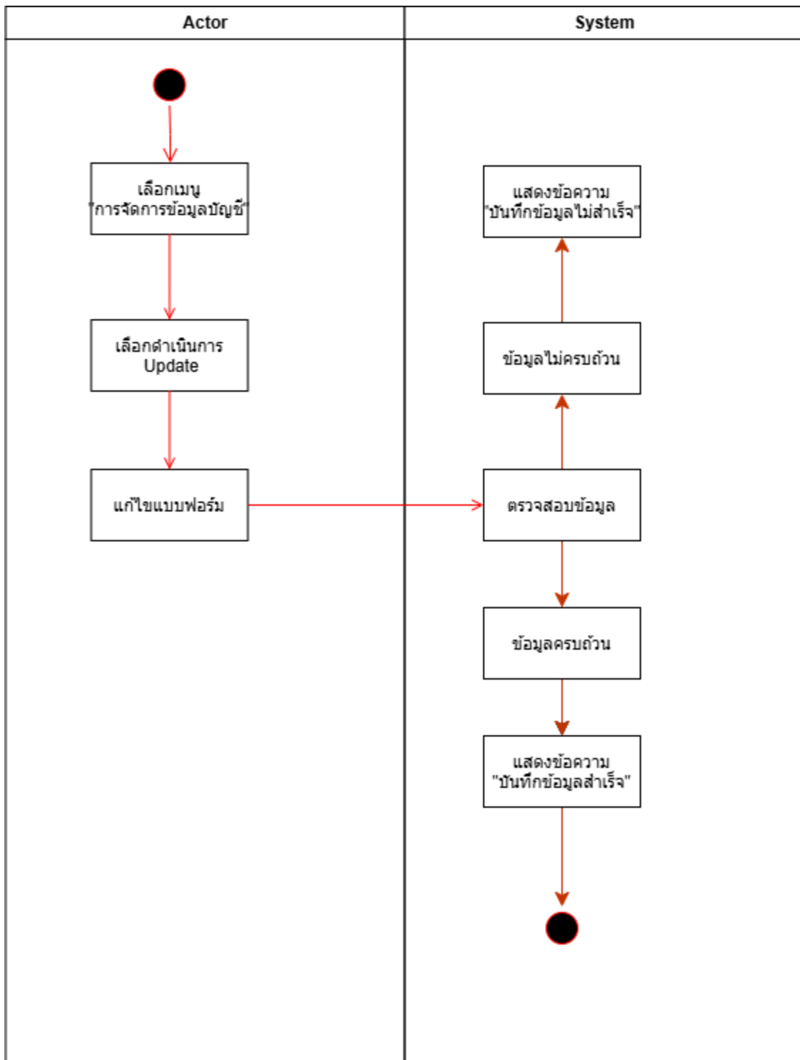
รูปภาพที่ 29 Activity Diagram (UC- 02 ) Update
