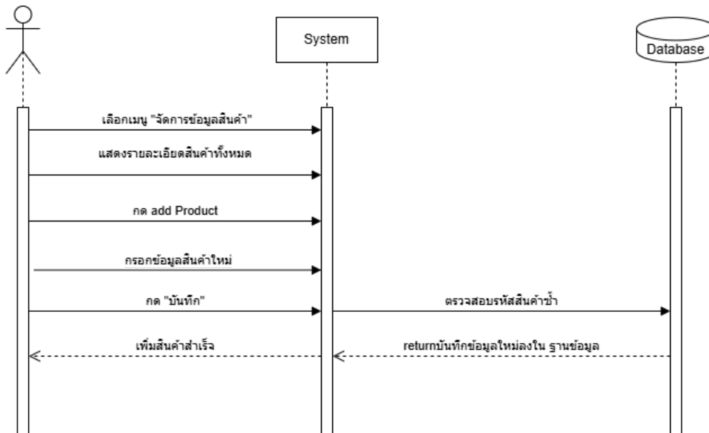
ภาพที่ 23 Sequence Diagram (UC-07) Manage product information(Add)
