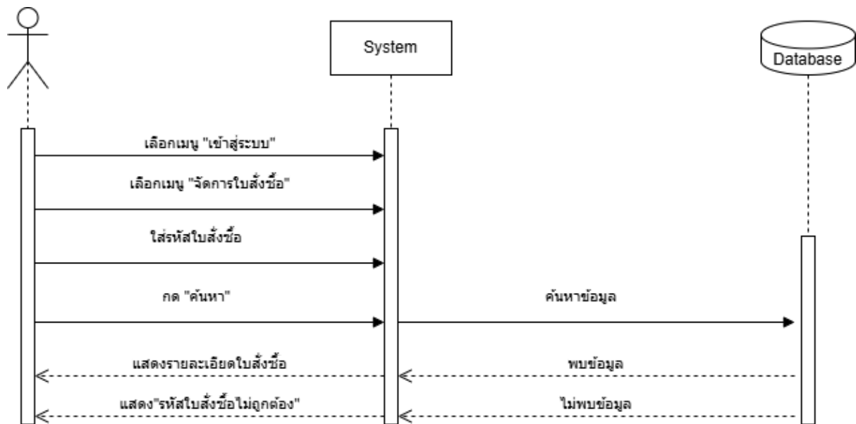
ภาพที่ 17 Sequence Diagram (UC-04) Manage purchase order information (Sale Officer)
