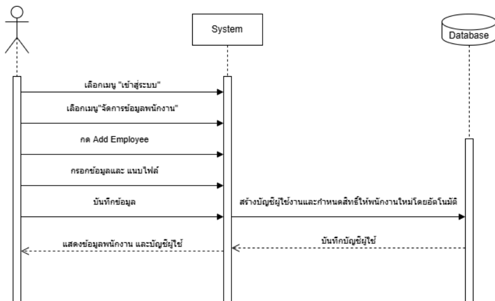
ภาพที่ 20 Sequence Diagram (UC-05) Manage Employee Information (Add)
