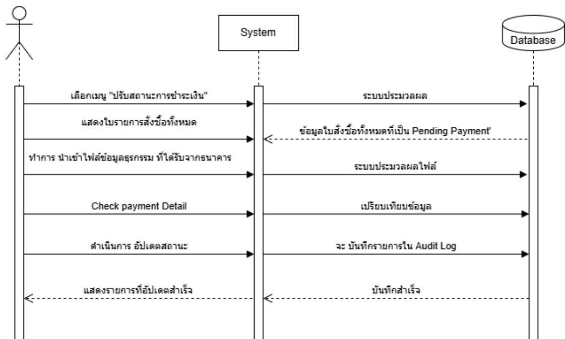
ภาพที่ 22 Sequence Diagram (UC-06) Adjust payment
