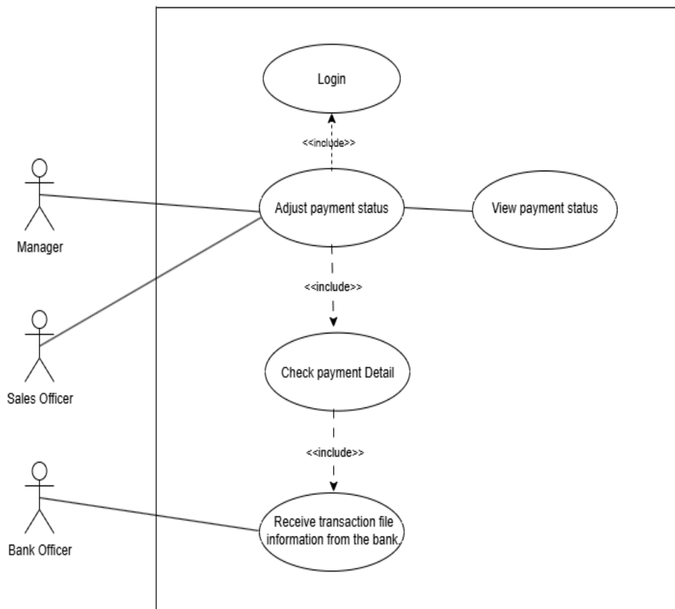
ภาพที่ 7 Use Case Diagram (UC- 06) Adjust payment status
