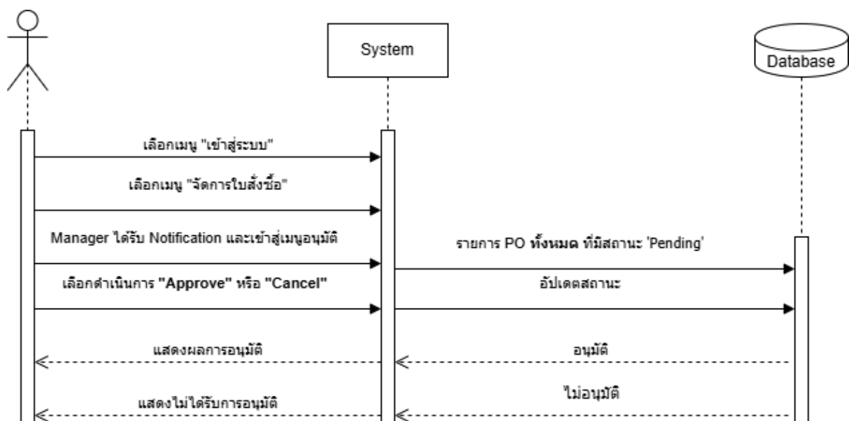
ภาพที่ 18 Sequence Diagram (UC-04) Manage purchase order information (Manager)
