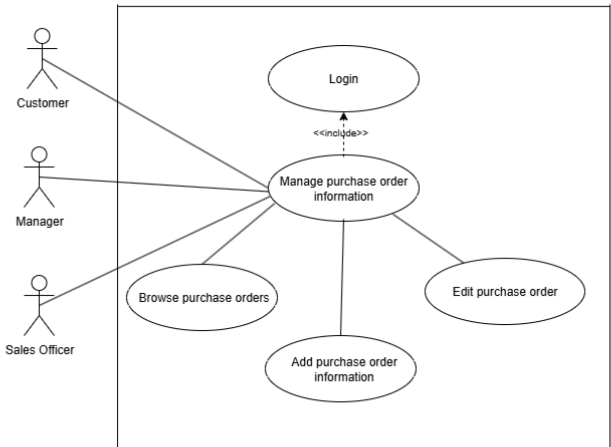
ภาพที่ 5 Use Case Diagram (UC- 04) Manage purchase order information
