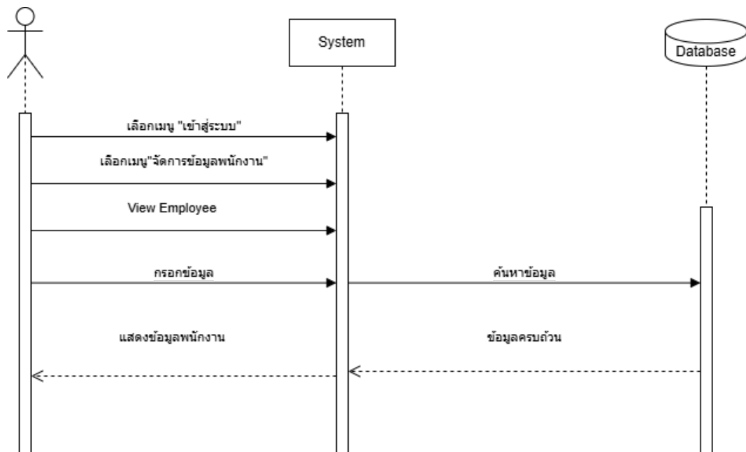
ภาพที่ 21 Sequence Diagram (UC-05) Manage Employee Information (View)
