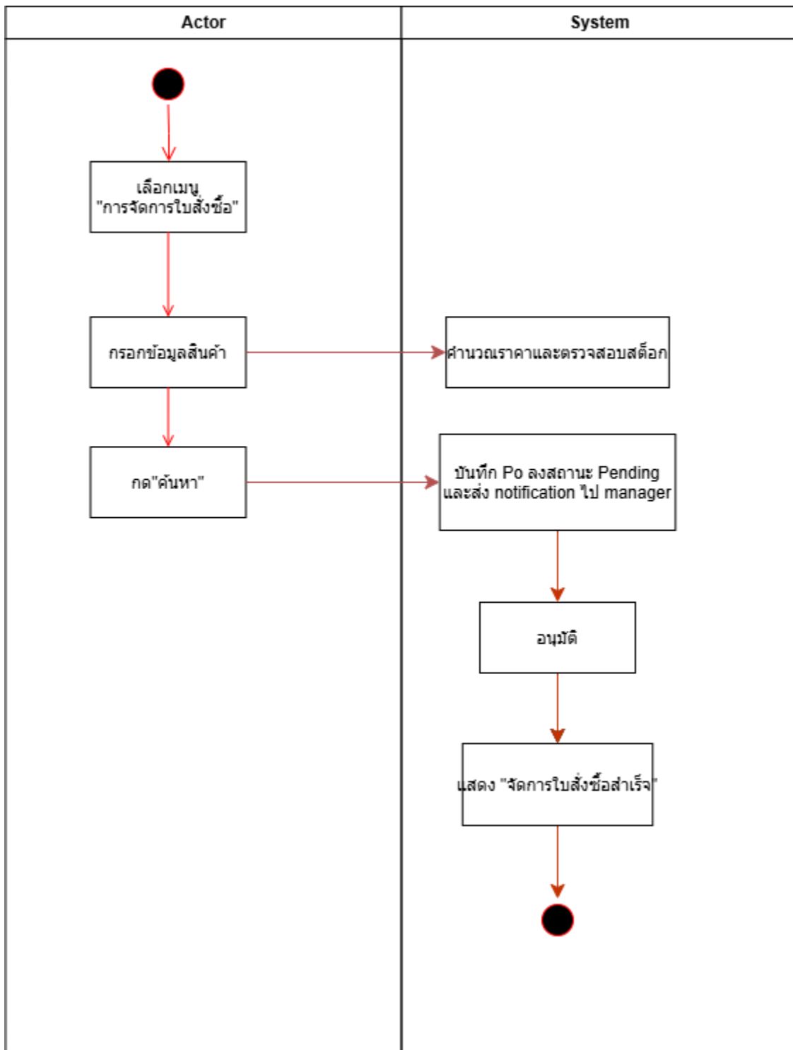
รูปภาพที่ 32 Activity Diagram (UC- 04 ) Manage purchase order information (customer)
