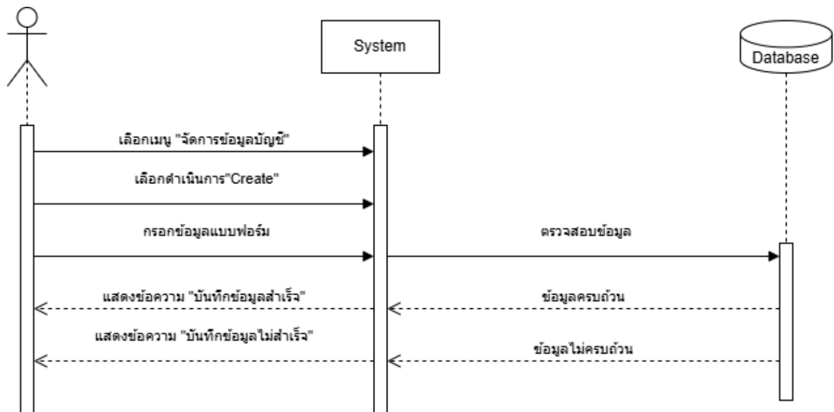
ภาพที่ 12 Sequence Diagram (UC-02) สร้างบัญชีผู้ใช้
