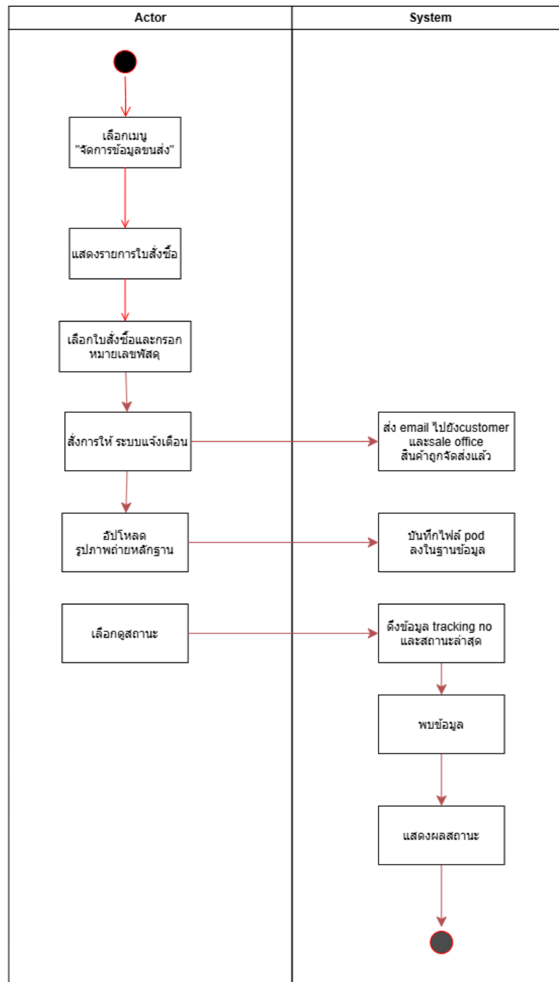
รูปภาพที่ 40 Activity Diagram (UC- 08 ) Get parcel delivery information and receipts
