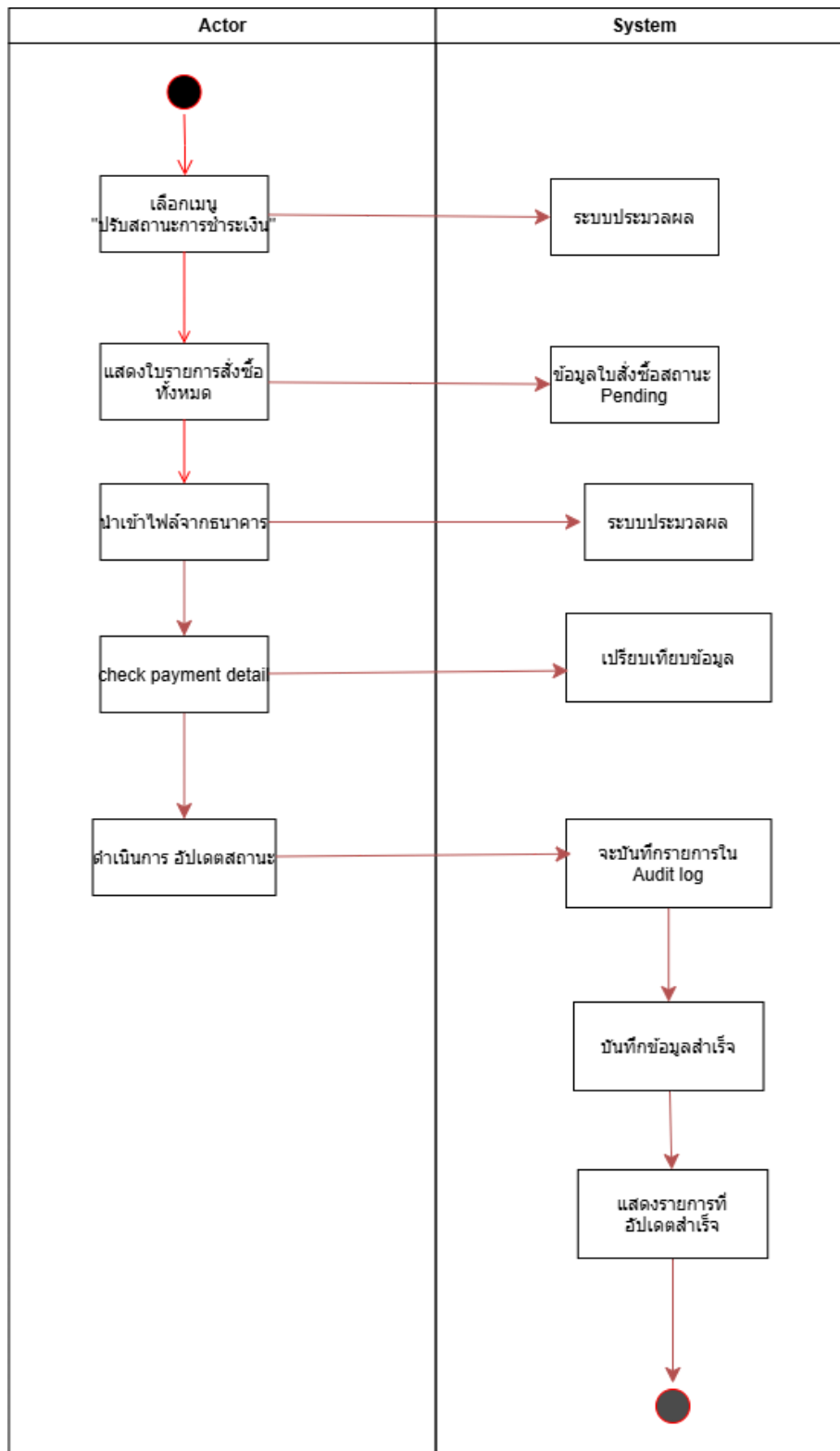
รูปภาพที่ 36 Activity Diagram (UC- 06 ) Adjust payment statusv(Manager ,Bank Office)
