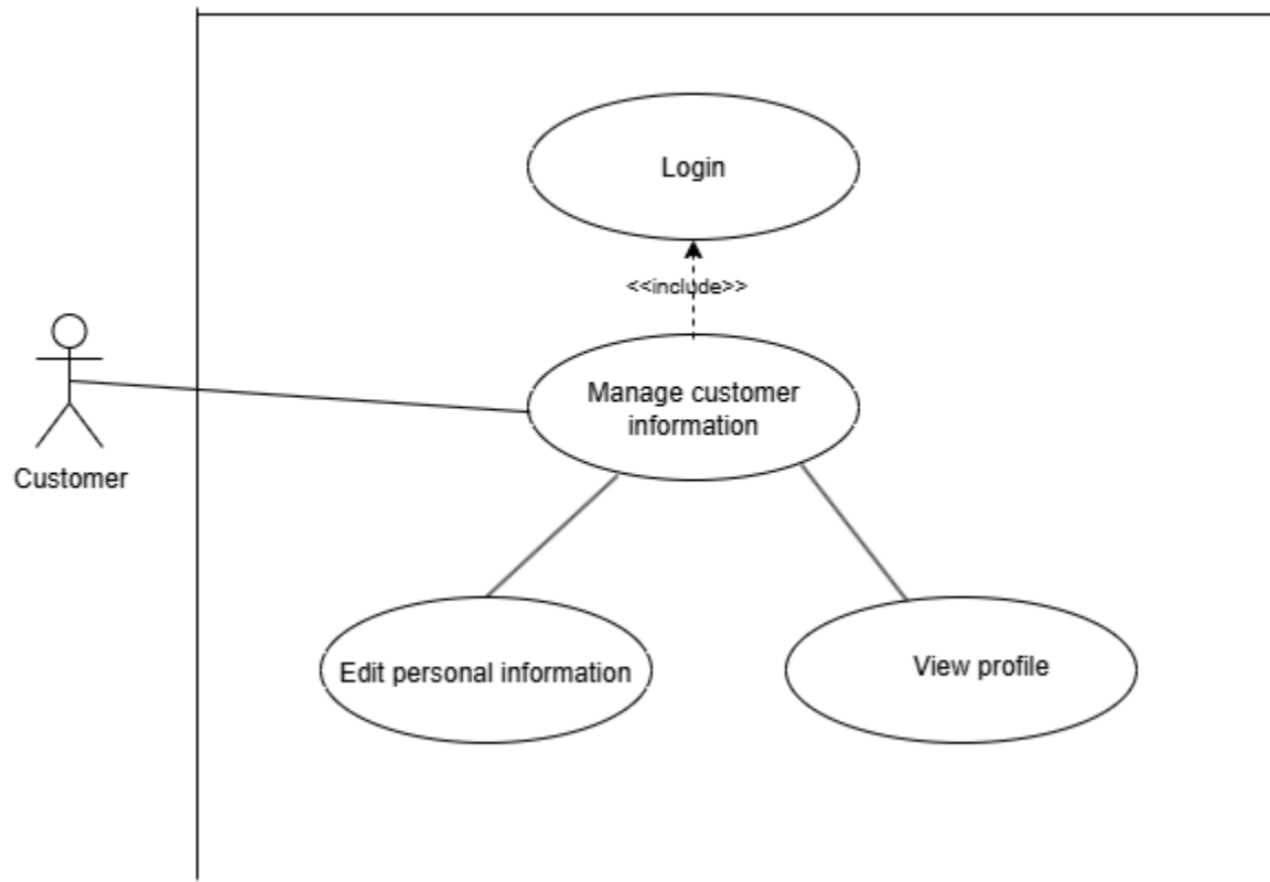
ภาพที่ 4 Use Case Diagram (UC- 03) Manage customer information
