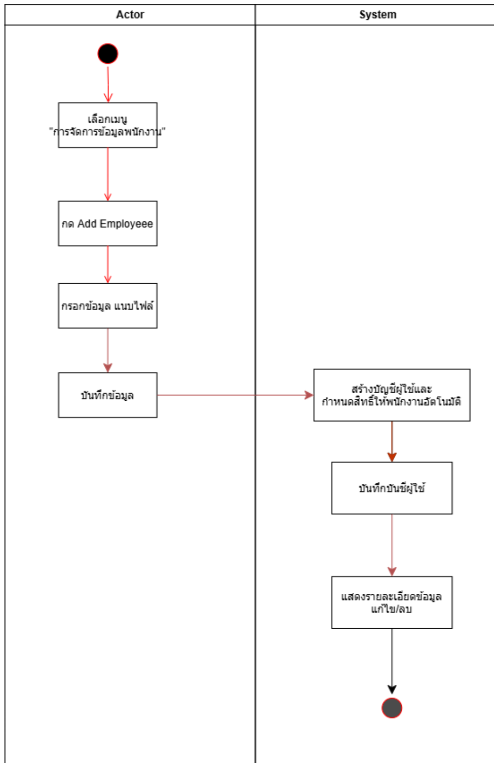
รูปภาพที่ 35 Activity Diagram (UC- 05 ) Manage Employee Information (Manager)
