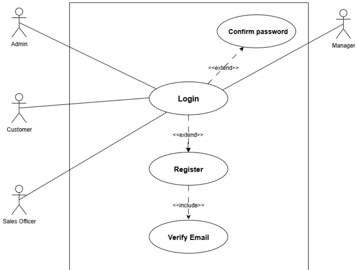
ภาพที่ 2 Use case Diagram (UC-01) Login
