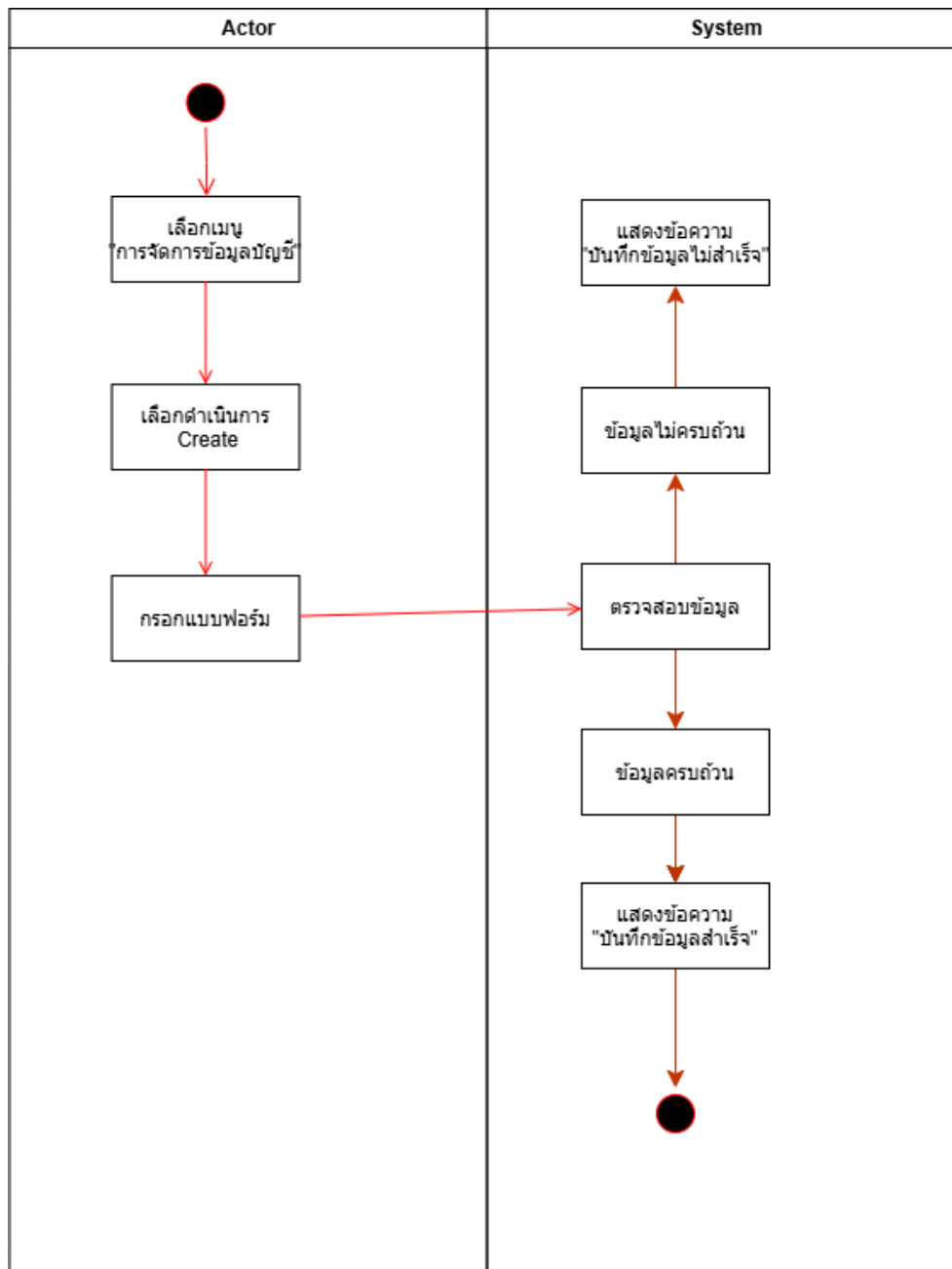
รูปภาพที่ 28 Activity Diagram (UC- 02 ) Create
