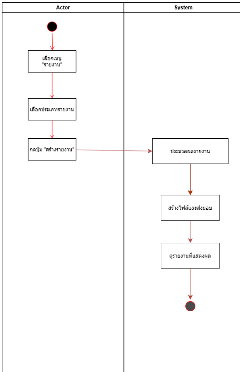
รูปภาพที่ 39 Activity Diagram (UC- 08 ) Process and Report Activity Diagram (UC- 09)
