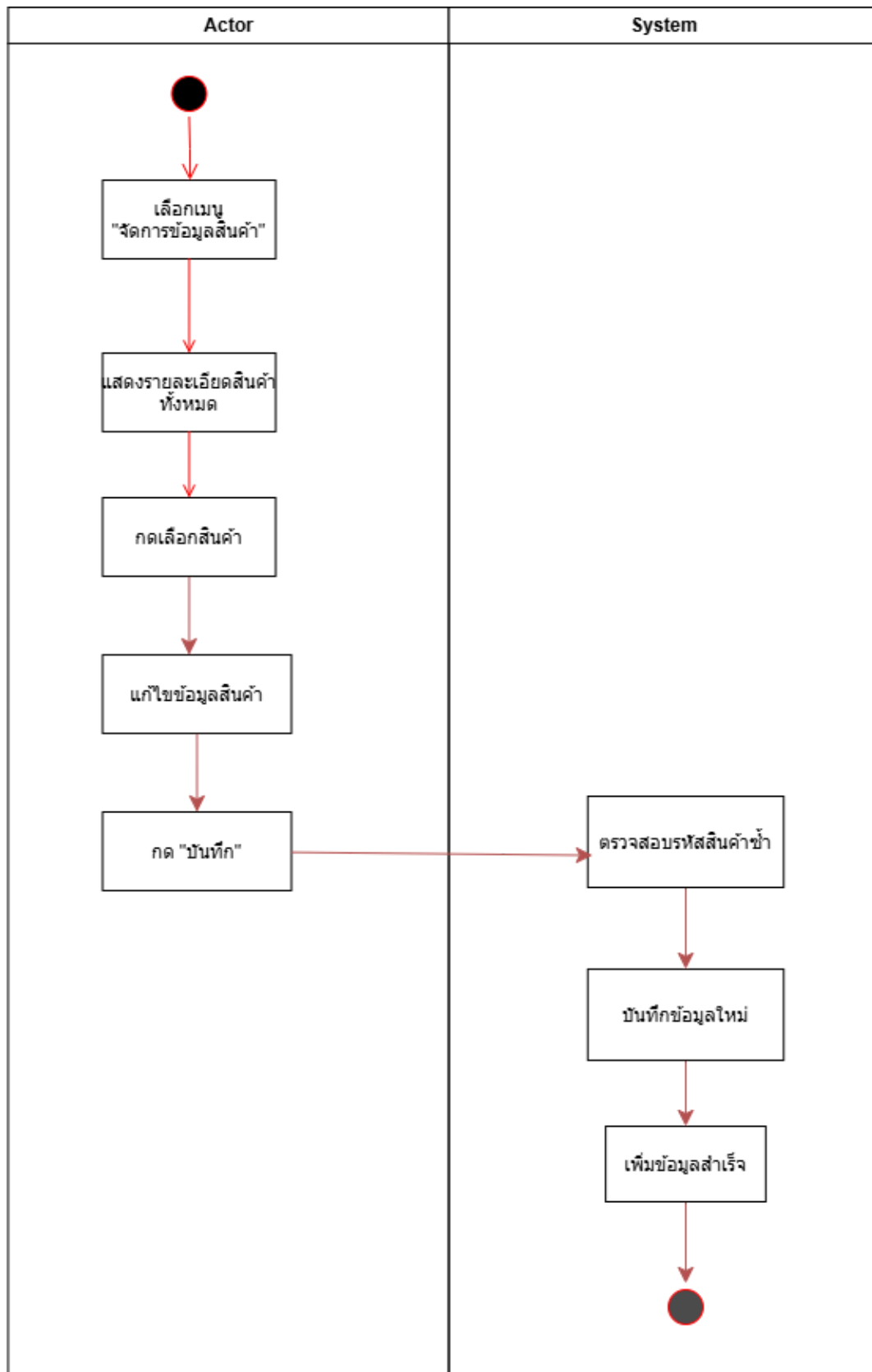
รูปภาพที่ 38 Activity Diagram (UC- 07) Manage product information(Update)
