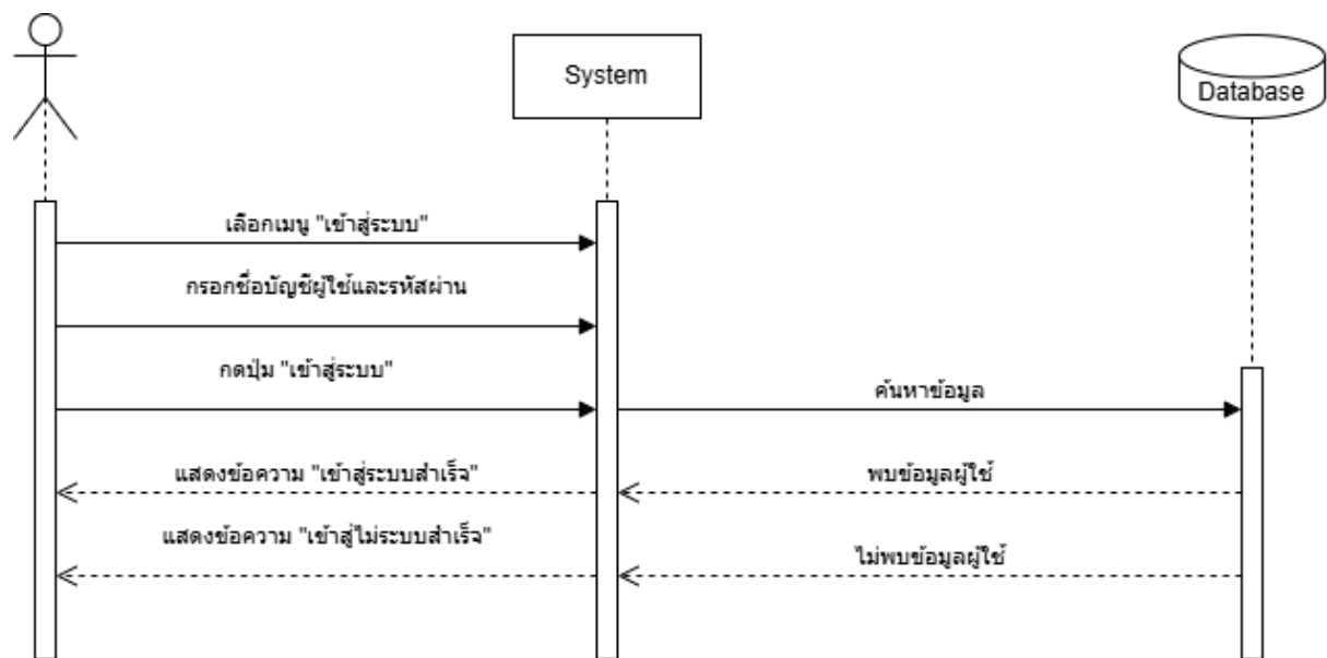
ภาพที่ 11 Sequence Diagram (UC-01) Login
