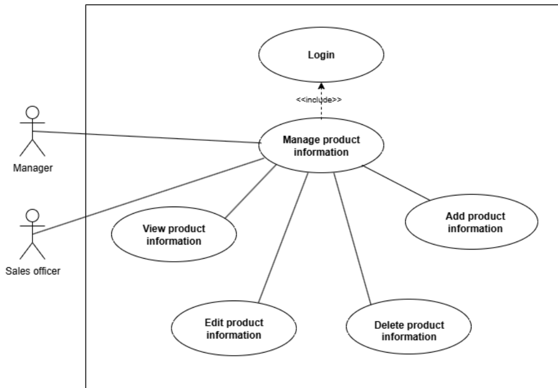
ภาพที่ 8 Use Case Diagram (UC- 07) Manage product information
