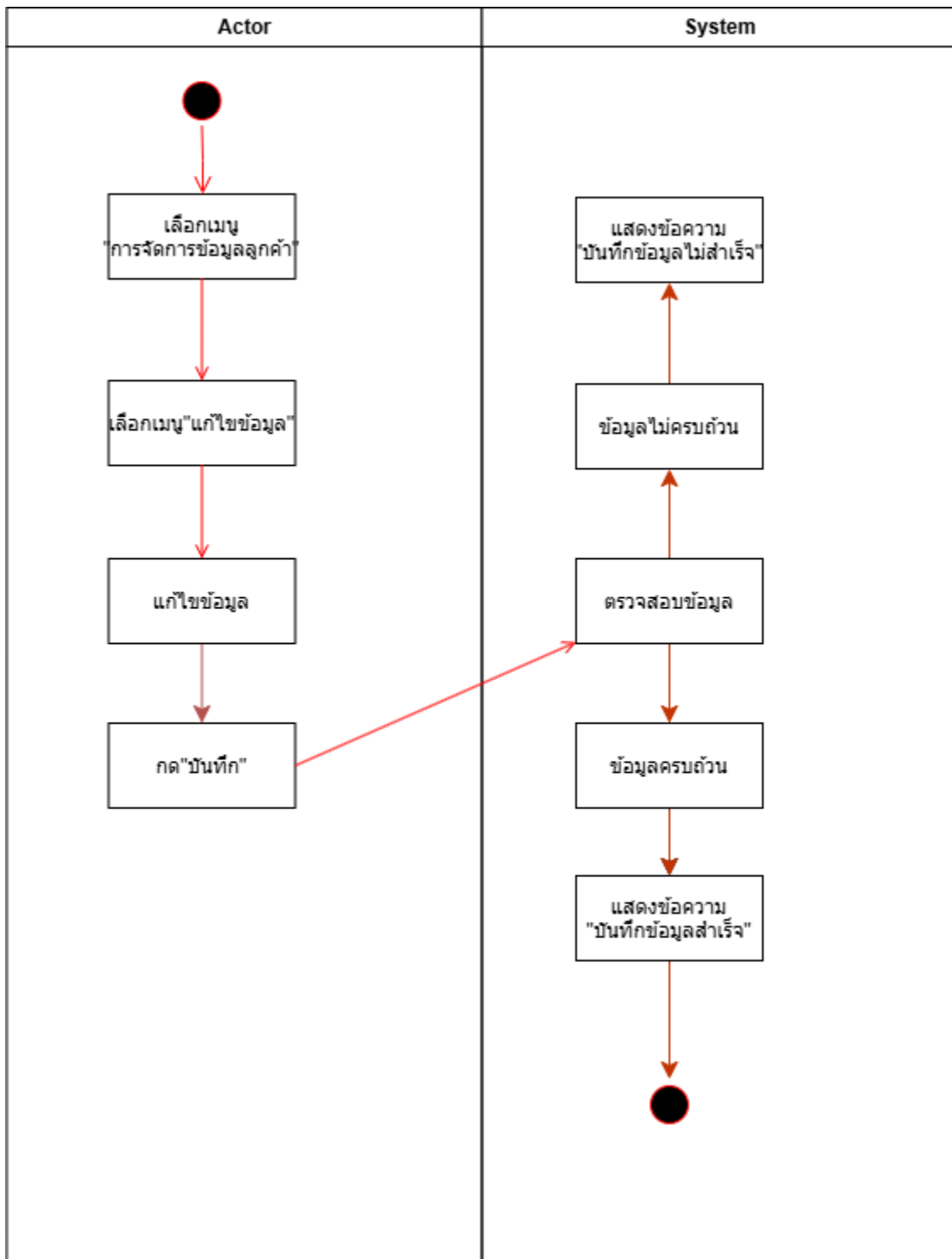
รูปภาพที่ 31 Activity Diagram (UC- 03 ) Manage customer information
