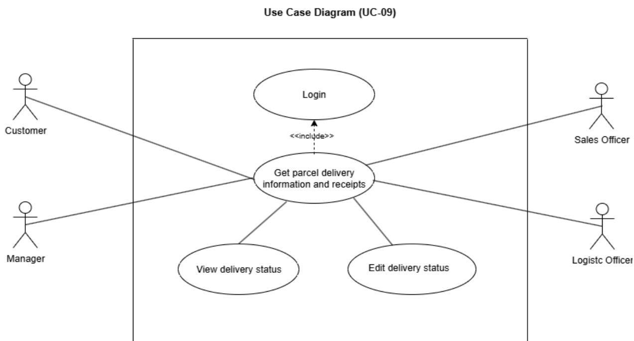
ภาพที่ 10 Use Case Diagram (UC- 09) Get parcel delivery information and receipts
