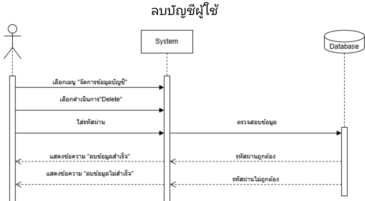
ภาพที่ 14 Sequence Diagram (UC-02) ลบบัญชีผู้ใช้
