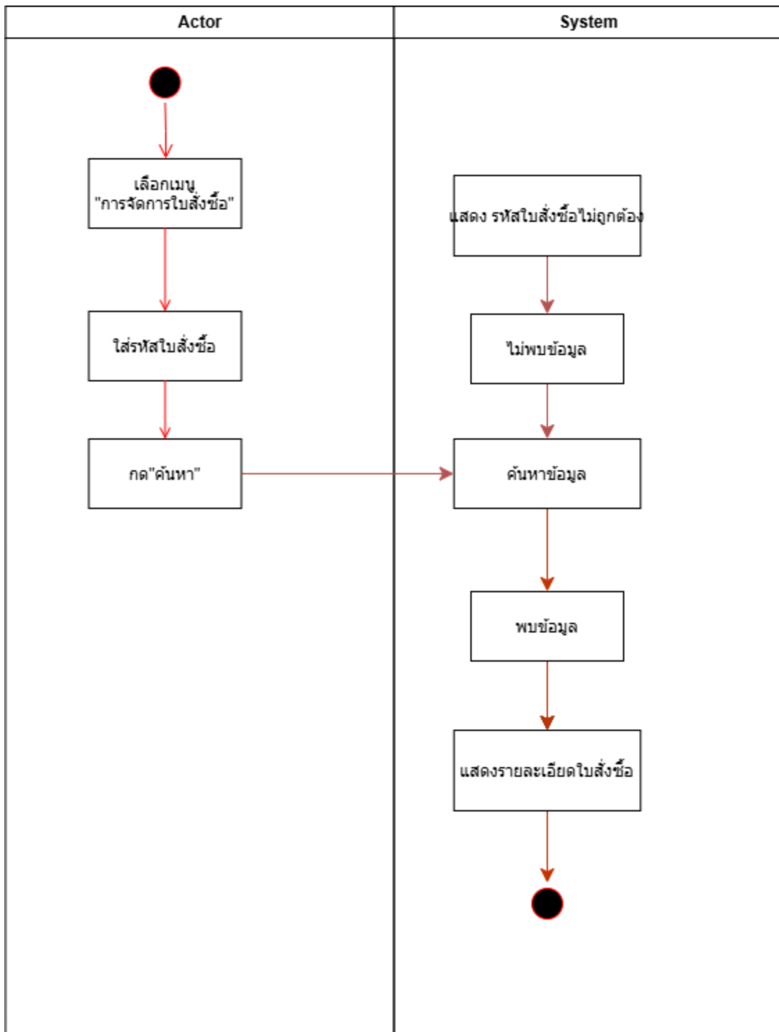
รูปภาพที่ 33 Activity Diagram (UC- 04) Manage purchase order information (Sale Officer)
