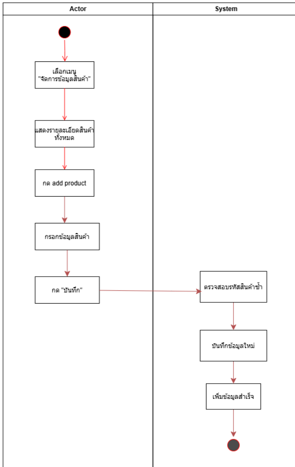
รูปภาพที่ 37 Activity Diagram (UC- 07 ) Manage product information(Add)
