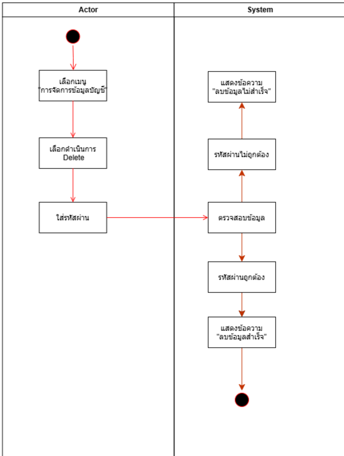
รูปภาพที่ 30 Activity Diagram (UC- 02 ) Delete
