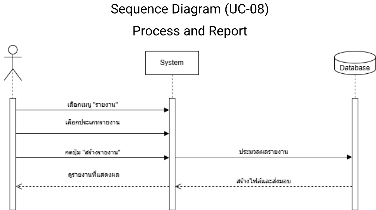
ภาพที่ 25 Sequence Diagram (UC-08) Process and Report
