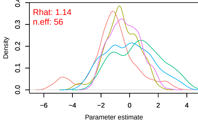
Density – alpha0[9]
