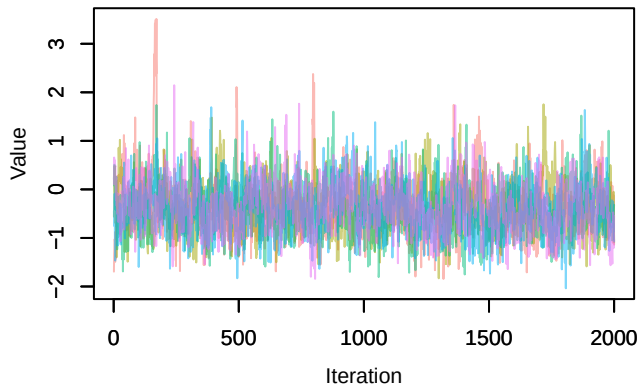
Trace – beta0[9]
