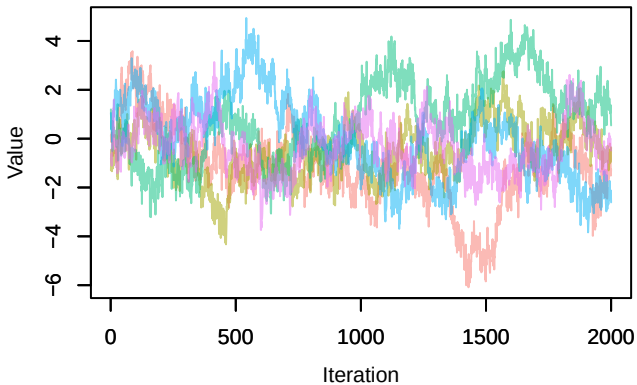
Trace – alpha0[9]
