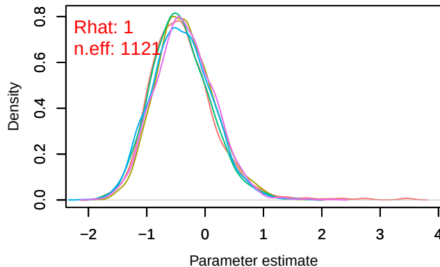
Density – beta0[9]
