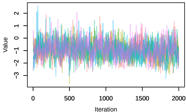
Trace – beta0[9]
