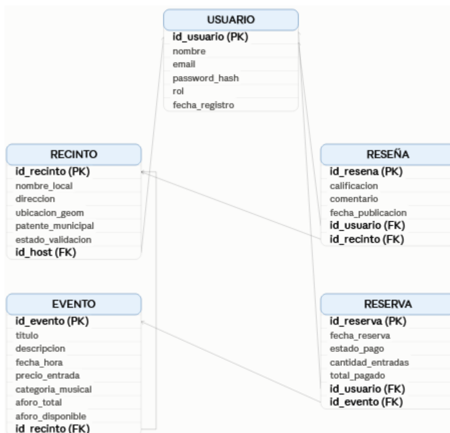
Figura 6: Esquema Relacional Lógico
