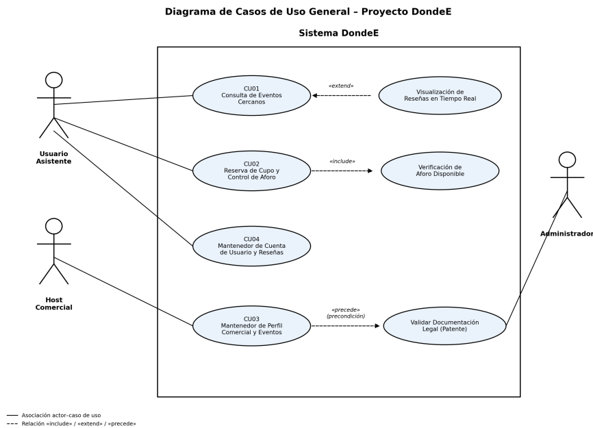
Figura 1: Diagrama de Casos de Uso General - Proyecto DondeE
