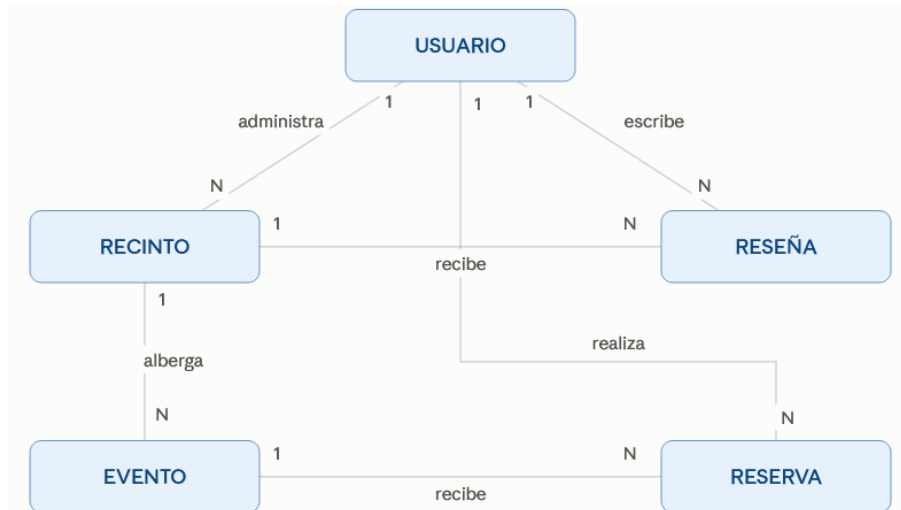
Figura 5: Modelo Entidad-Relación Conceptual
