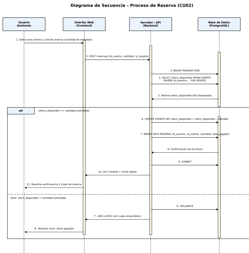
Figura 2: Diagrama de Secuencia Propuesto - Flujo Transaccional Esperado
