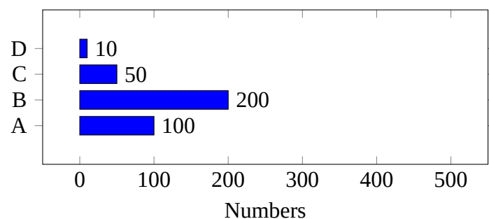
圖 3.3 A barchart.
