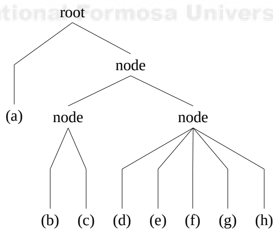
圖 3.2 A tree.
