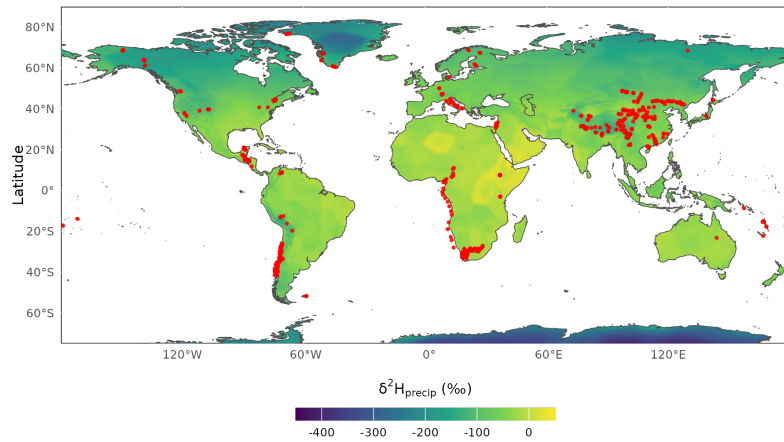
A: \delta^2\text{H} precipitation
