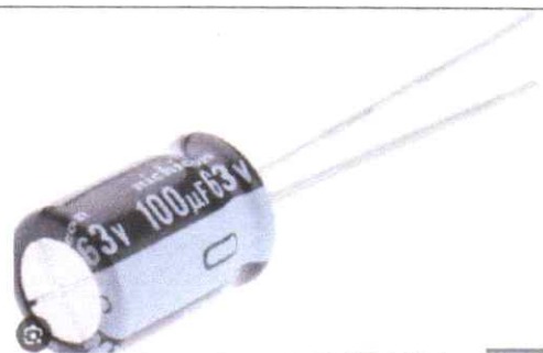
Kapasitor 100MF 63V
