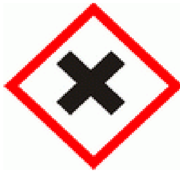
Gambar 6. Simbol B3 klasifikasi bersifat berbahaya ( harmful )
