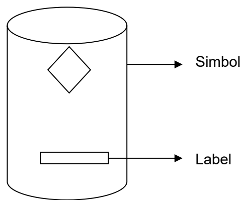
Gambar 13. Kemasan B3 dengan simbol dan label
