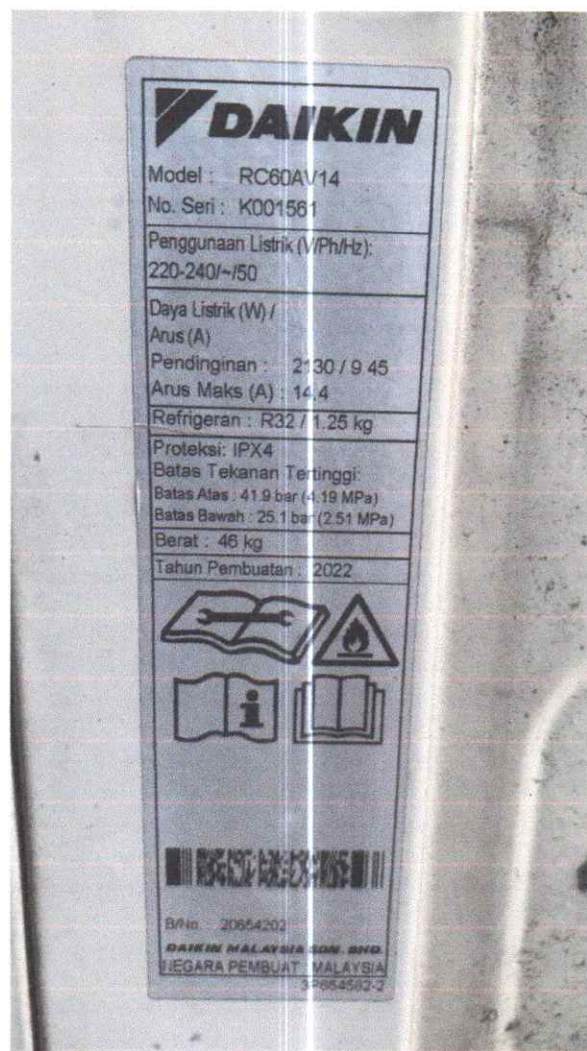
Kompresor 2,5 PK Rotary Merk Daikin Freon R32
