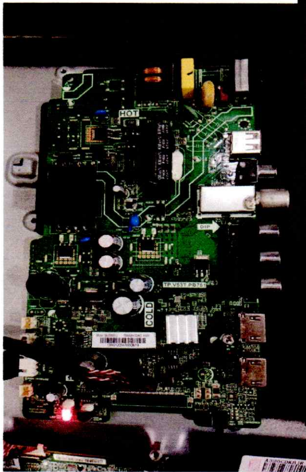
Modul dan Lampu Backlight
