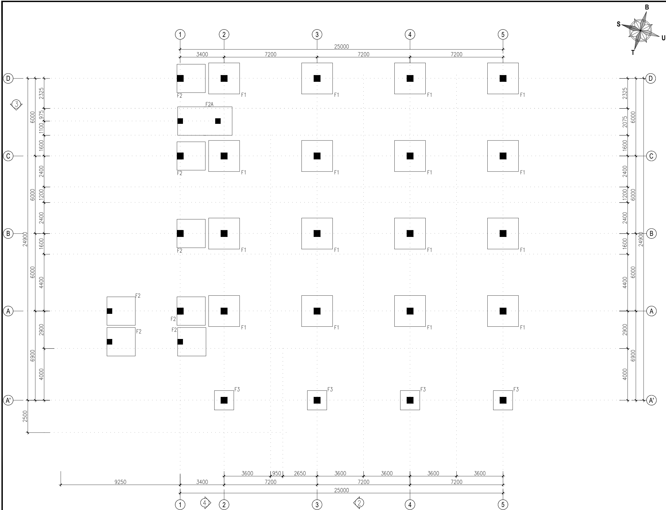
STR DENAH PONDASI SKALA 1 : 150
