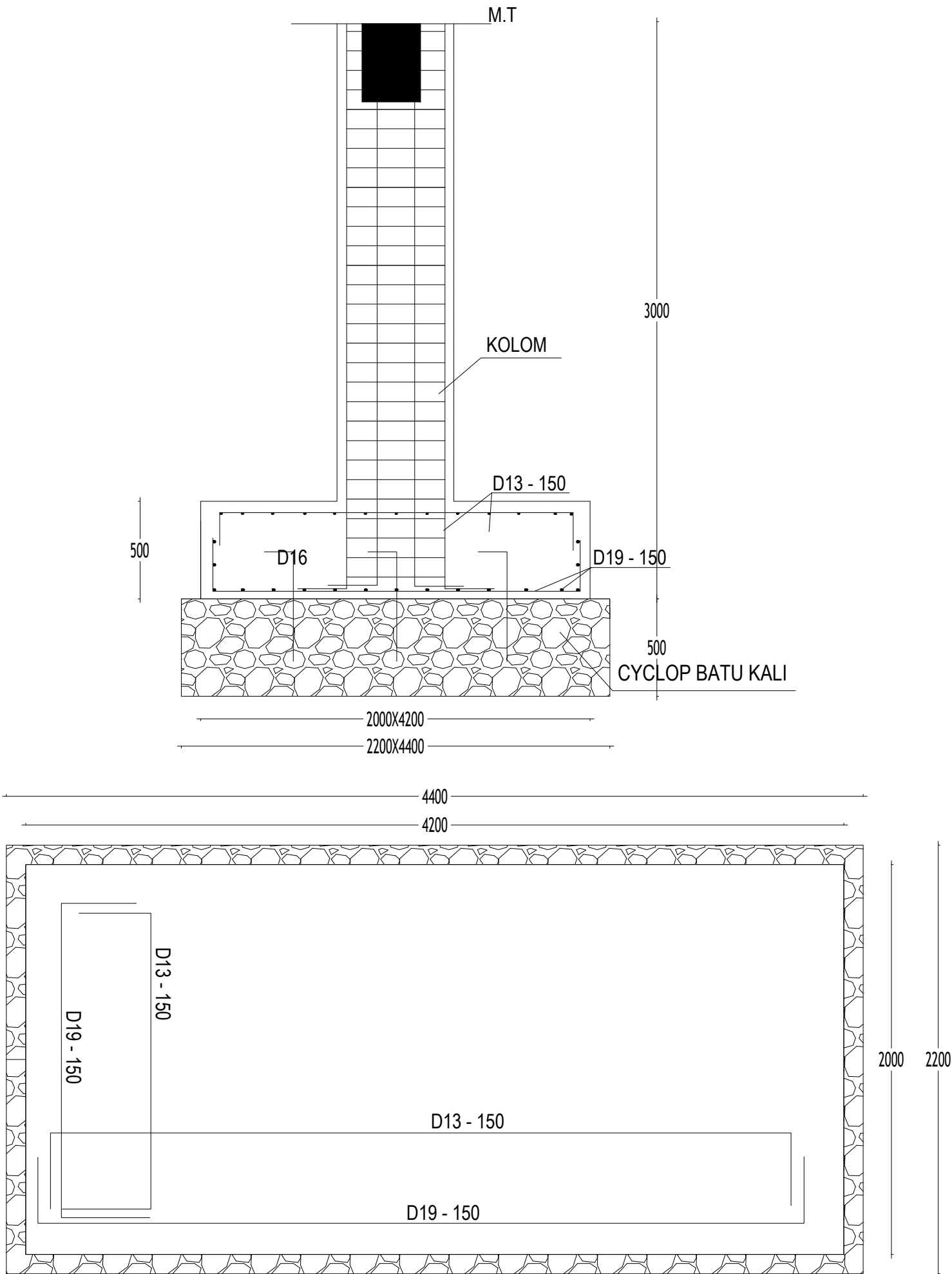
DETAIL FONDASI F2A
