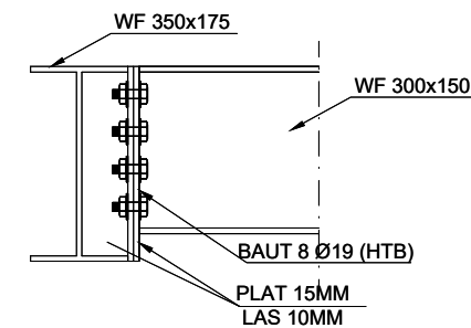
DETIL B3 KE B2 SKALA 1 : 15
