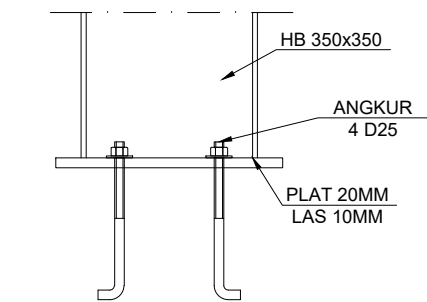
DETIL KOLOM K1 HB 350x350 SKALA 1 : 15
