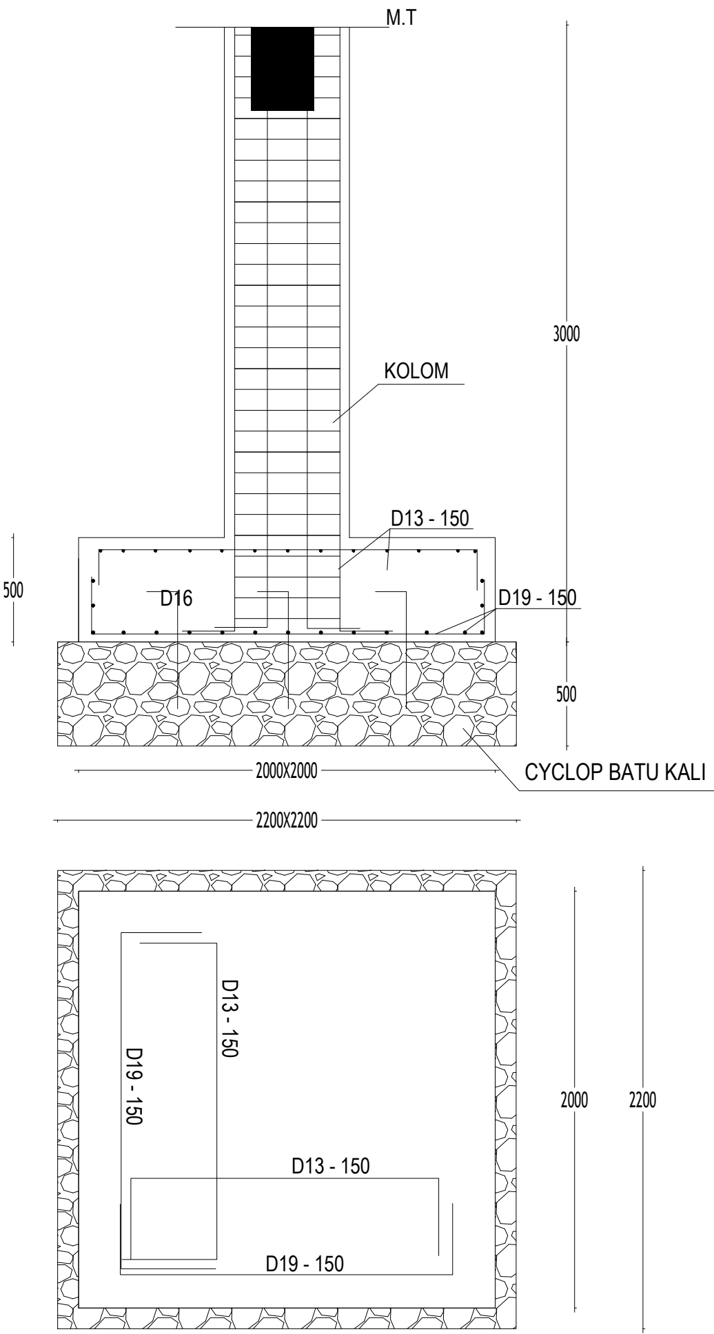
DETAIL FONDASI F2
