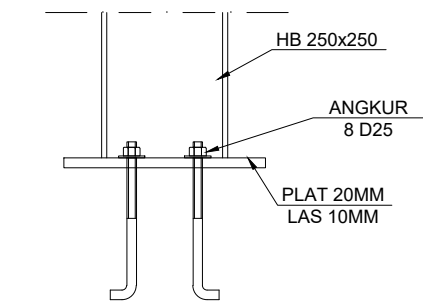
DETIL KOLOM K2 HB 250x250 SKALA 1 : 15
