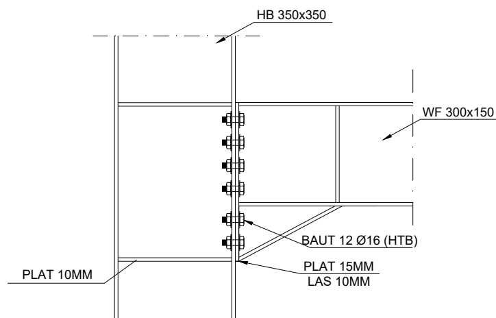
DETIL B3 KE KOLOM SKALA 1 : 15
