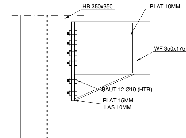
DETIL B2 KE KOLOM SKALA 1 : 15
