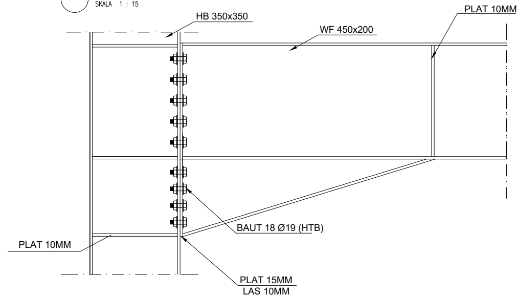
DETIL B1 KE KOLOM SKALA 1 : 15
