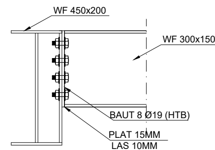
DETIL B3 KE B1 SKALA 1 : 15
