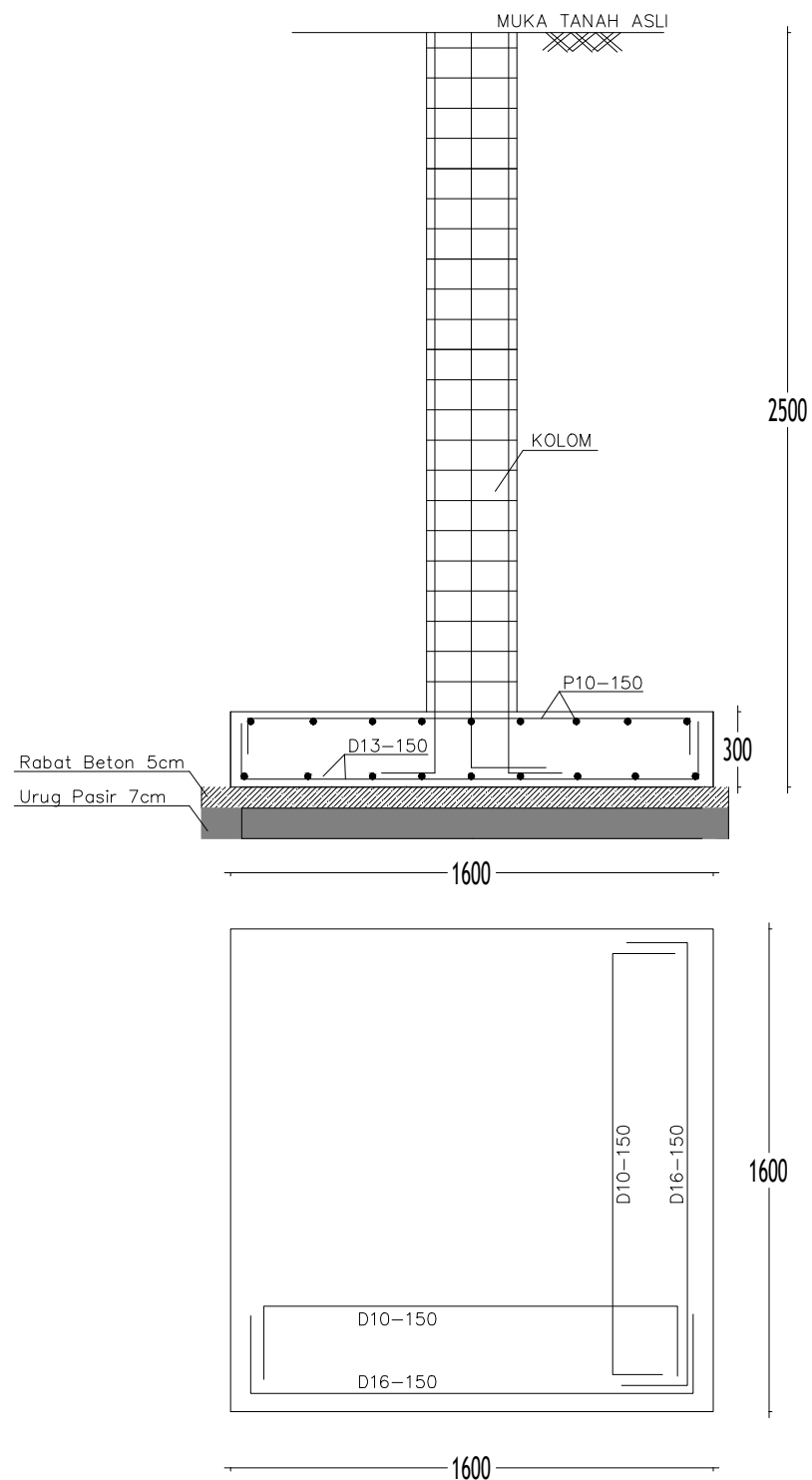
DETAIL FONDASI F3
